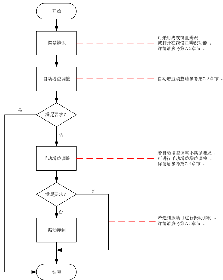
图 7-2 增益调整流程
