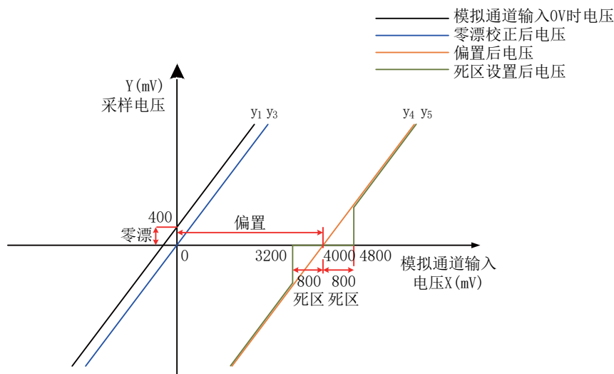
图 6-69 伺服驱动器 AI 处理对应采样电压举例
