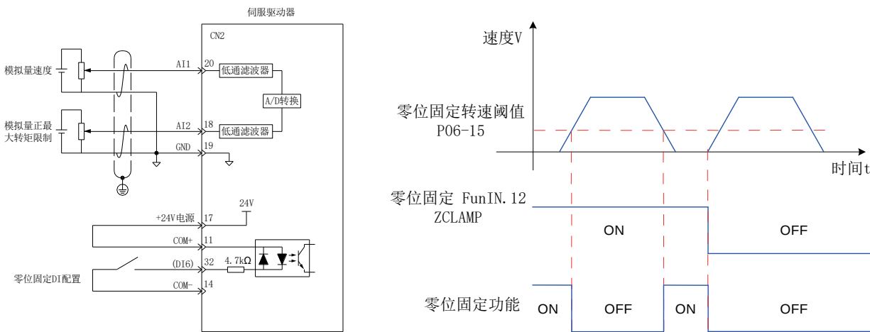
图 6-77 零位固定相关配线与波形图
