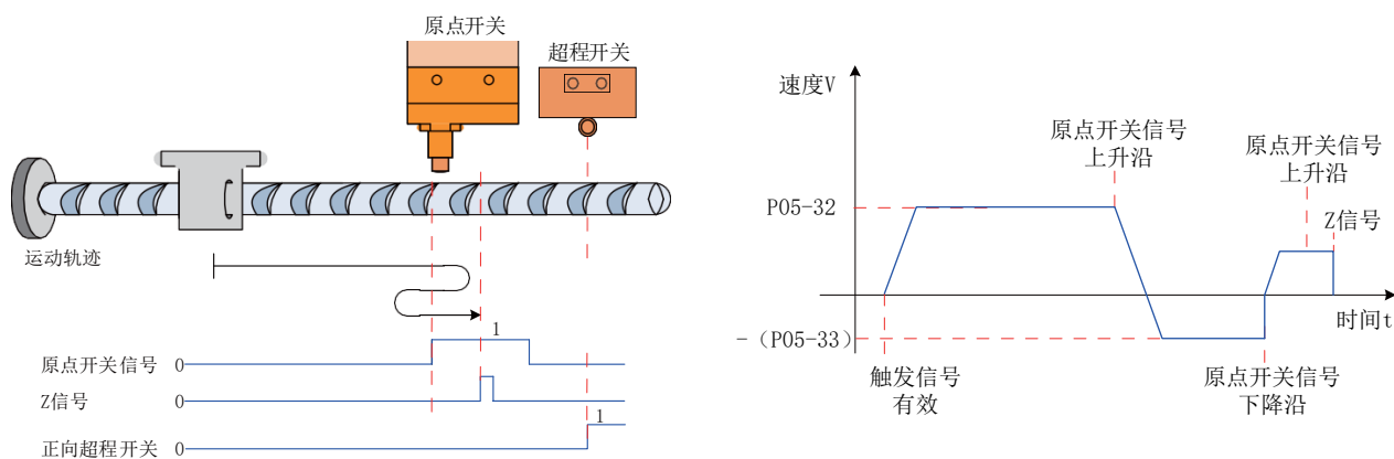
图 6-52 模式 4 原点回零电机运行曲线①与转速说明
