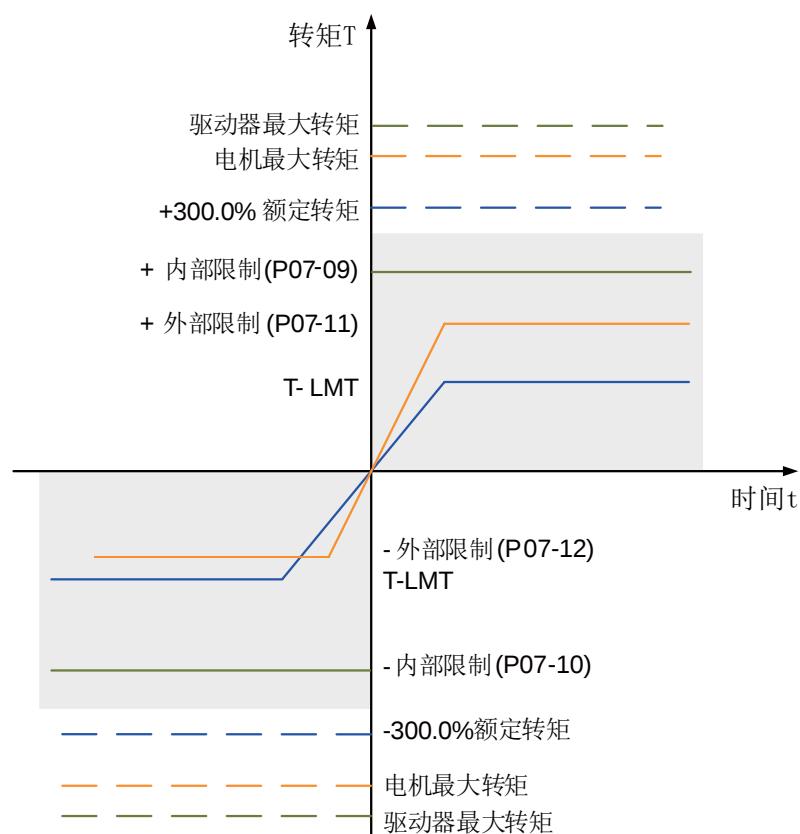
图 6-95 转矩限制举例
