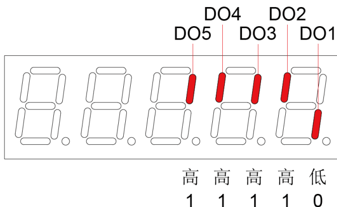
图 5-14 D0 端子电平均为“高电平有效”时 P0B-05 显示
