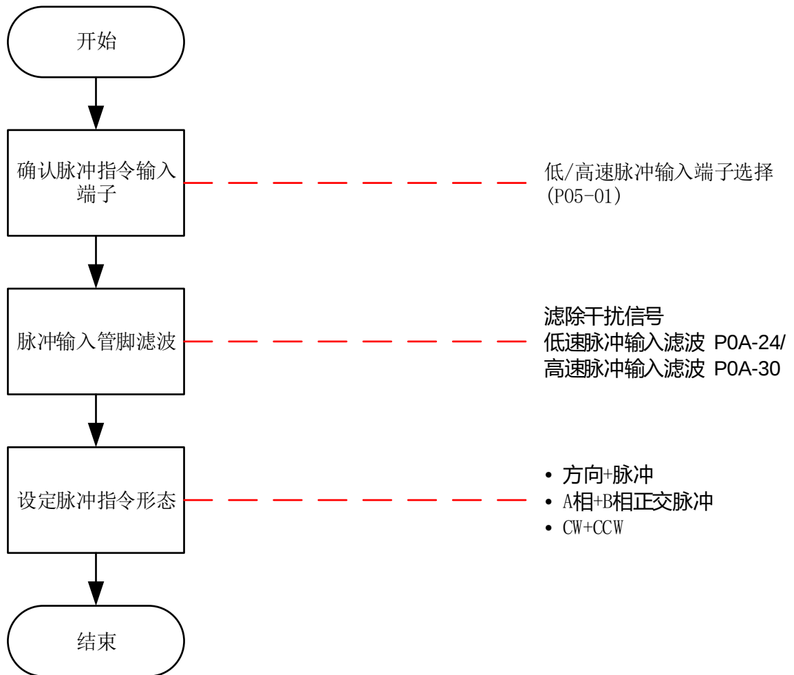
图 6-25 脉冲指令来源设置流程
