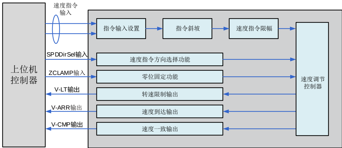
图 6-64 伺服驱动器与上位机信号交互图
