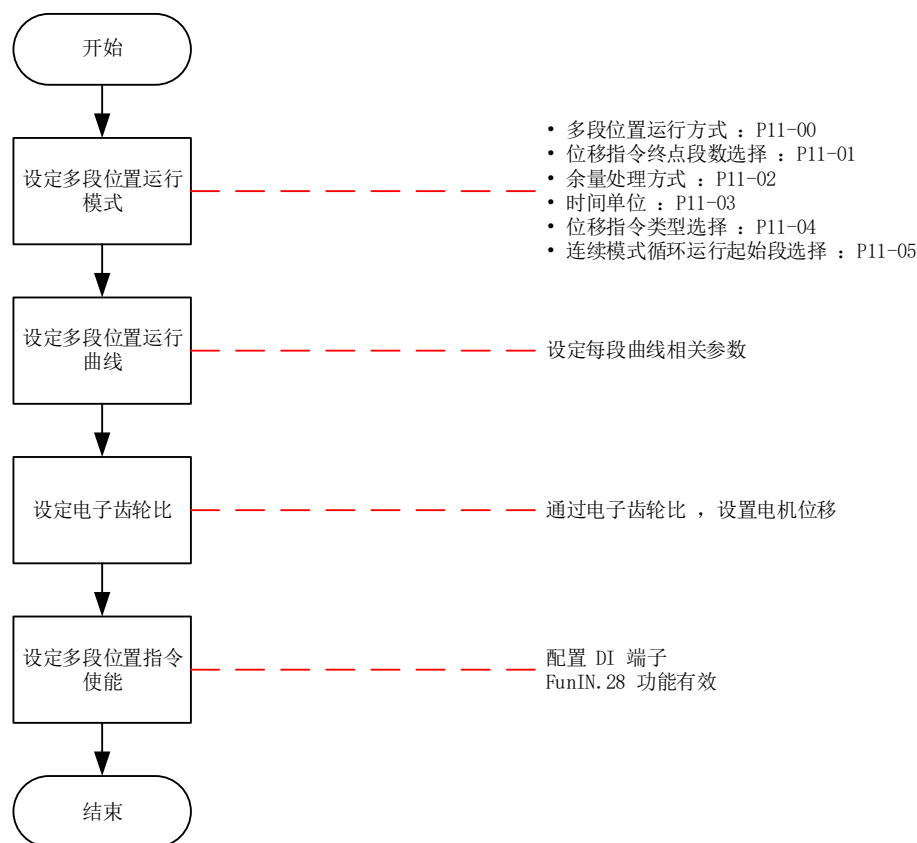
图 6-29 多段位置指令来源设置流程
