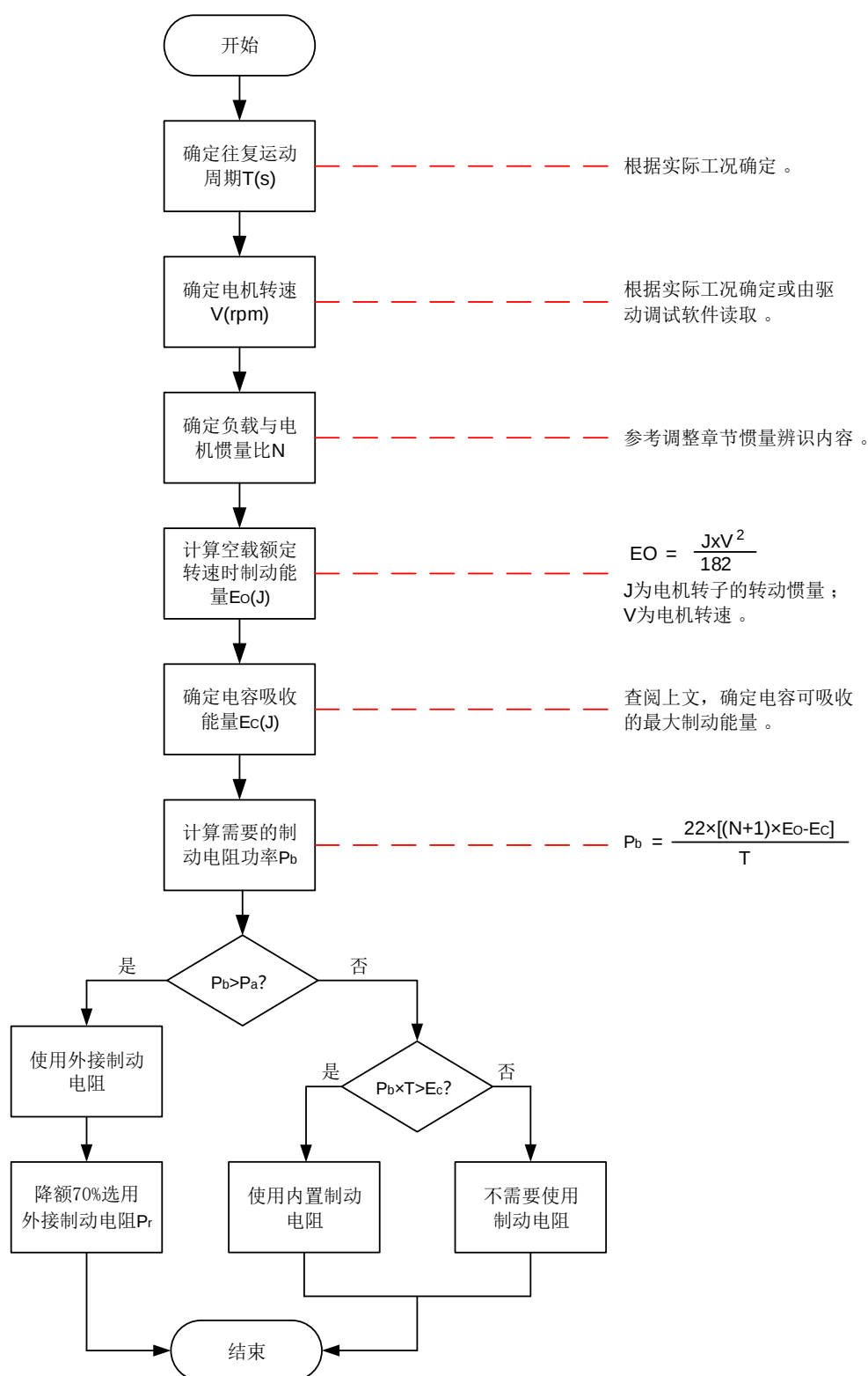
图6-8 制动电阻选型流程图
