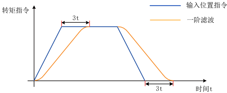
图 6-93 梯形转矩指令一阶滤波示意图
