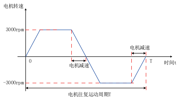
图6-7 外部负载转矩不存在情况下电机速度曲线举例
