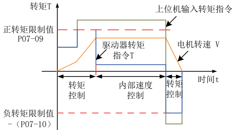
图 6-97 P07-07=0 转矩限制曲线图
