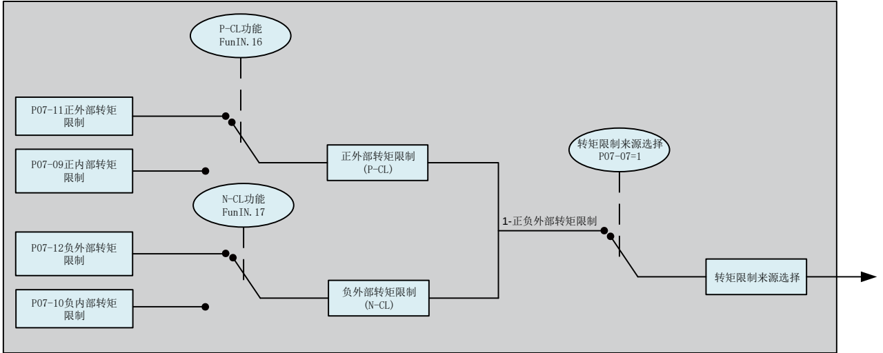
图 6-98 P07-07=1 转矩限制来源
