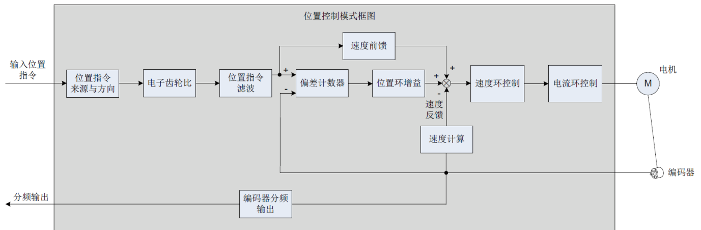
图 6-21 位置控制框图
