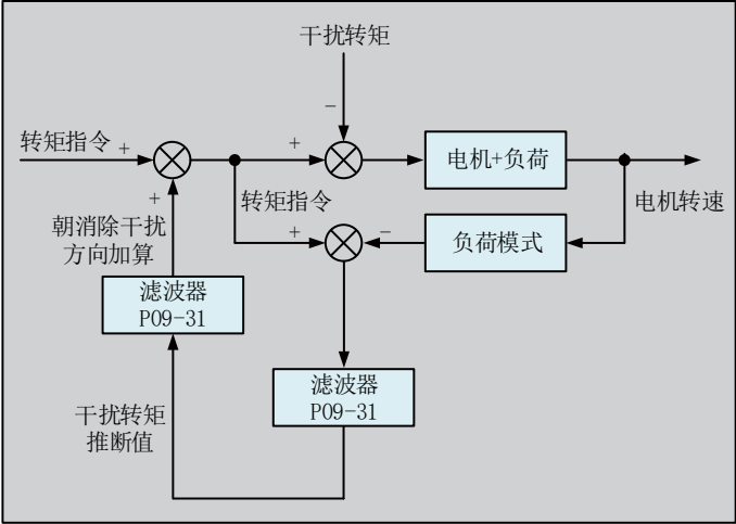
图 7-12 扰动观测功能框图
