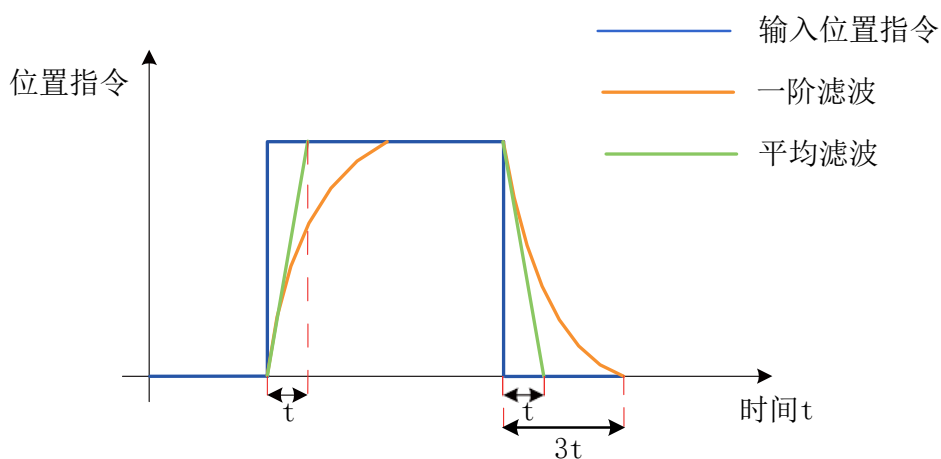
图6-38 矩形位置指令一阶滤波与平均滤波示意图
