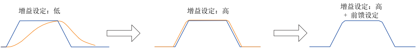
图 7-1 增益设定举例
