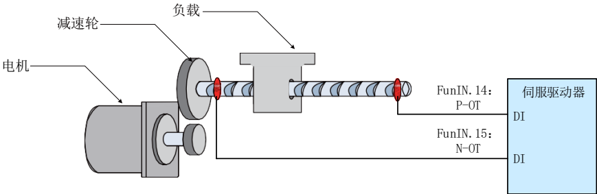
图 6-114 限位开关的安装示意图
