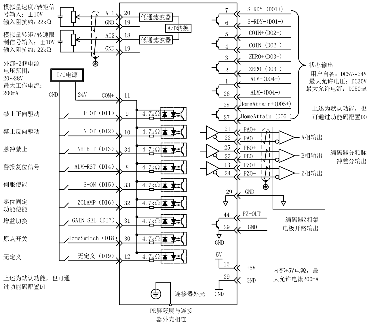
图 4-30 转矩模式配线图
