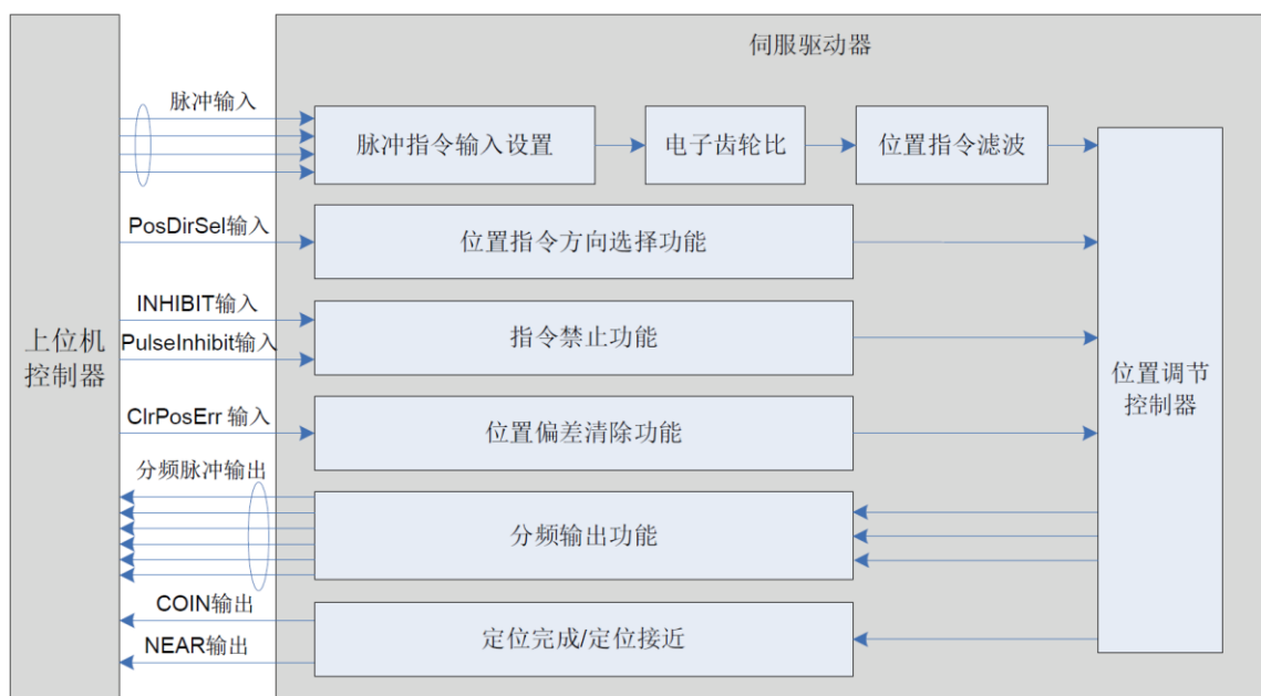
图 6-22 伺服驱动器与上位机信号交互图
