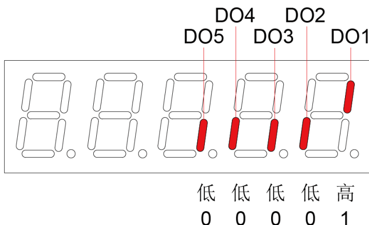
图 5-13 D0 端子电平均为“低电平有效”时 P0B-05 显示
