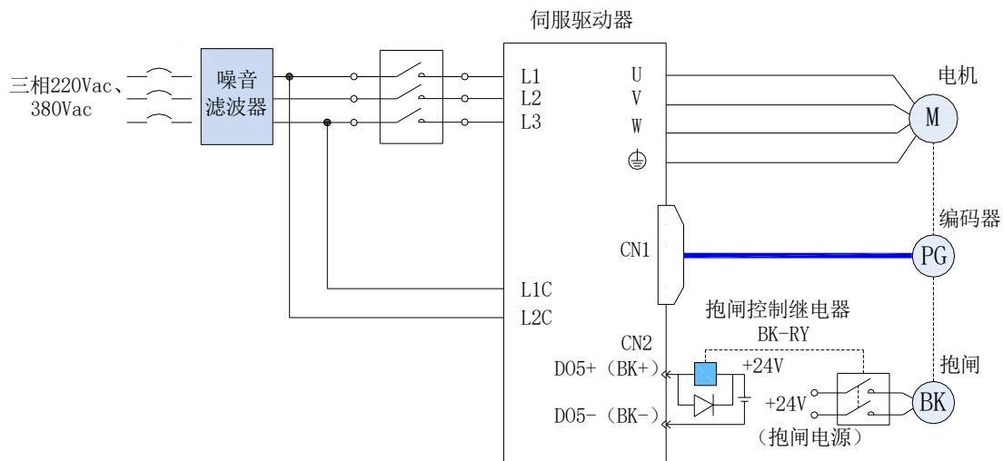
图4-10 抱闸配线图
