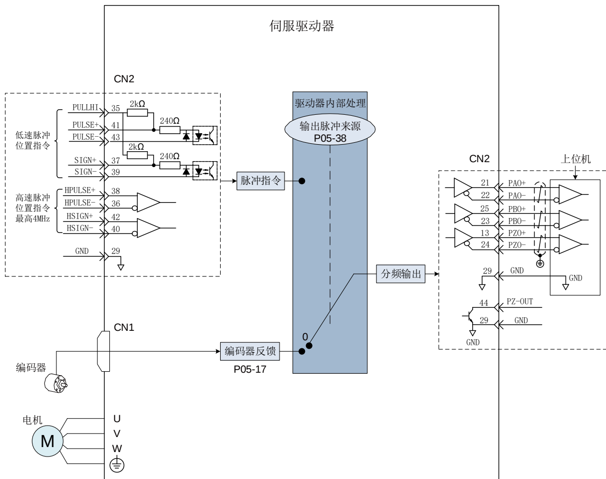
图 6-40 分频输出原理示意图
