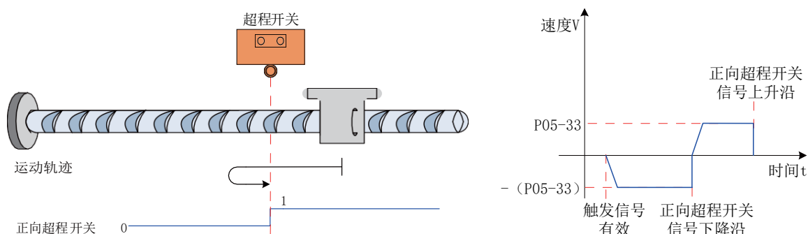
图 6-56 模式 6 原点回零电机运行曲线②与转速说明
