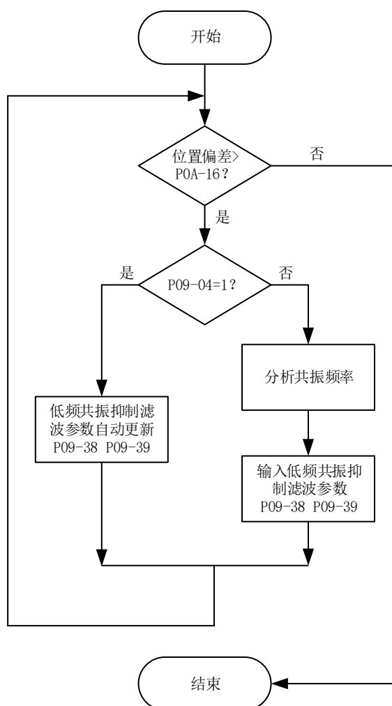
图 7-17 低频共振抑制滤波器使用步骤
