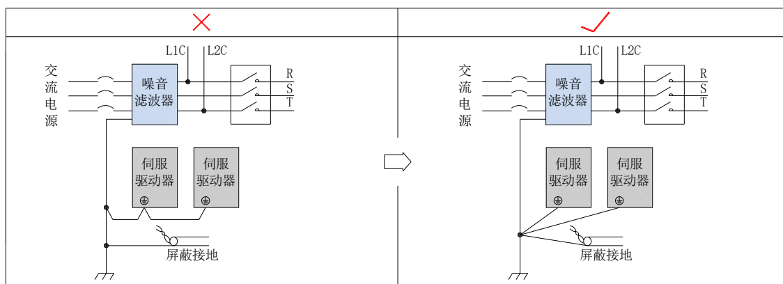
图 4-25 单点接地示意图
