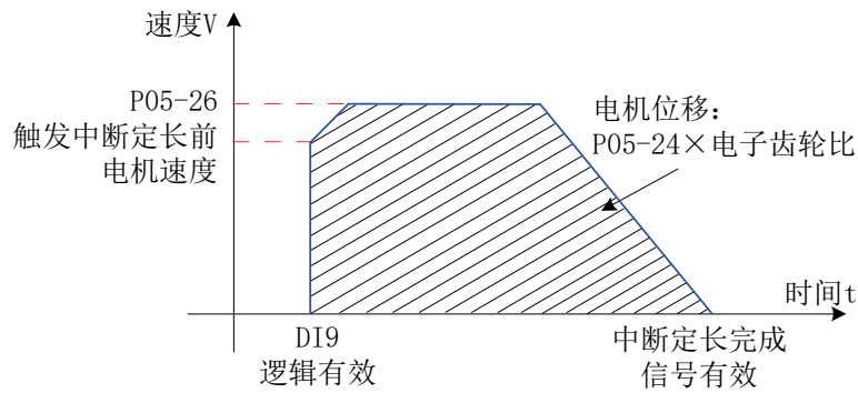
图 6-45 中断定长功能电机运行曲线
