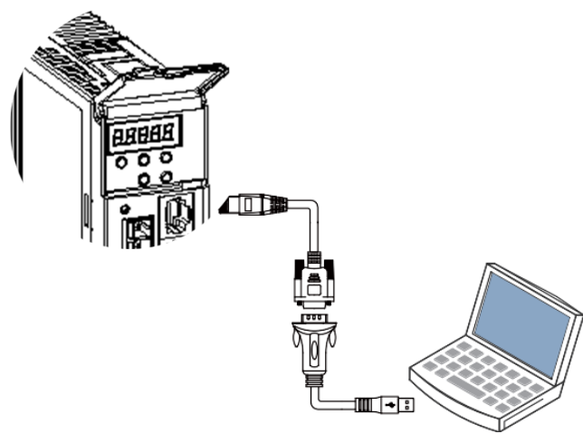
图4-21 通信串口转USB示意图
