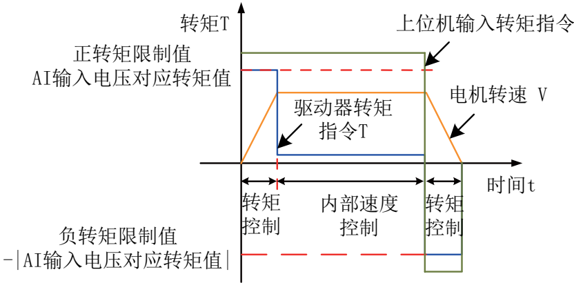
图 6-100 P07-07=2 转矩限制曲线图
