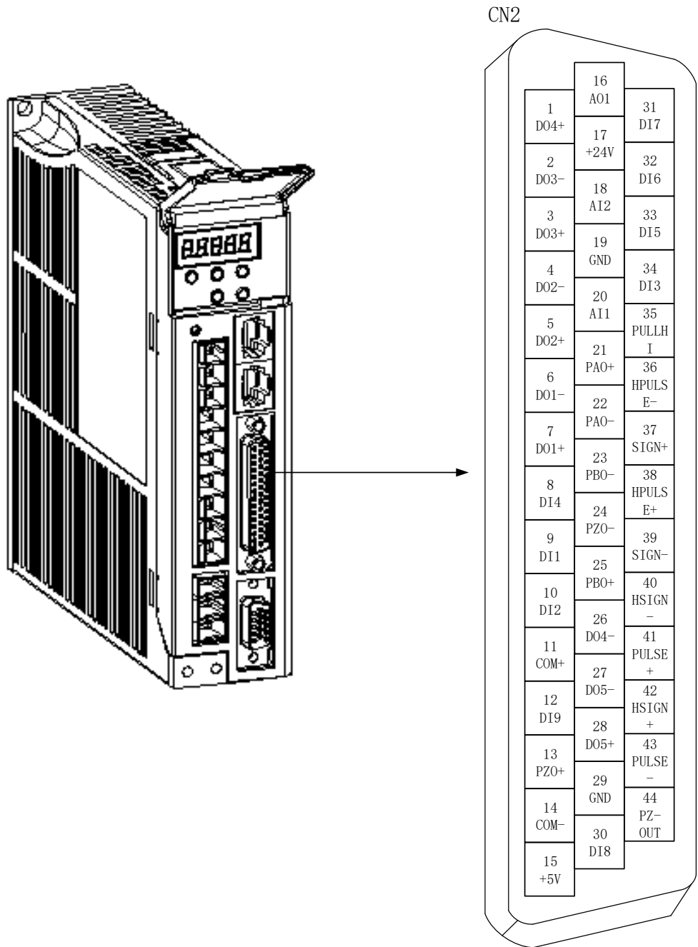
图4-8 驱动器控制回路端子连接器引脚分布图
