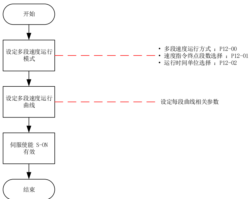
图 6-73 多段速度设置流程图
