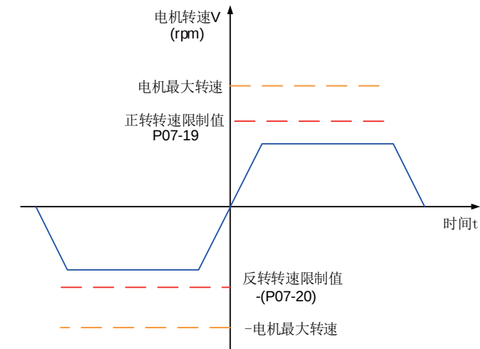
图 6-105 P07-17=0 速度限制曲线图
