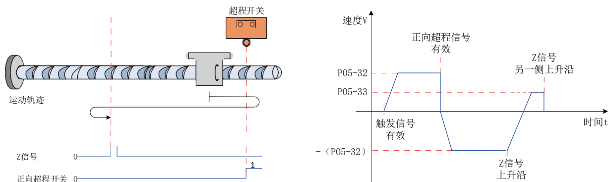
图 6-51 模式 2 原点回零电机运行曲线③与转速说明
