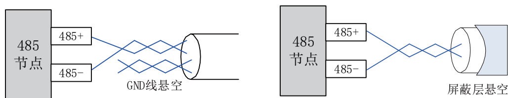
图10-11 无GND时的接线示意图
