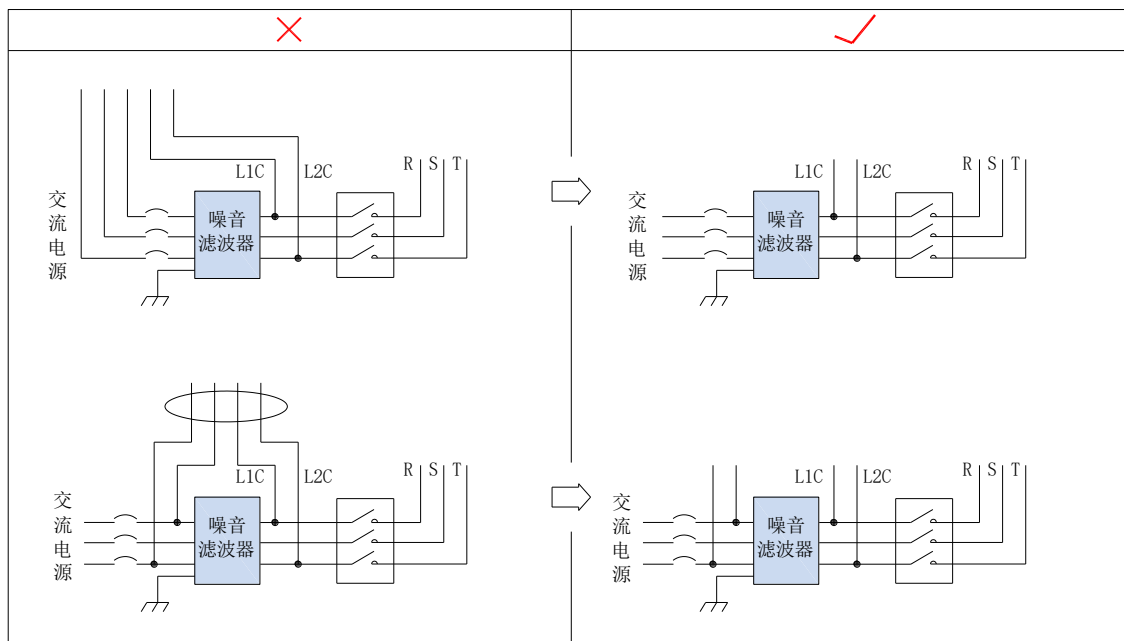
图4-23 噪音滤波器输入与输出配线分离走线示意图
