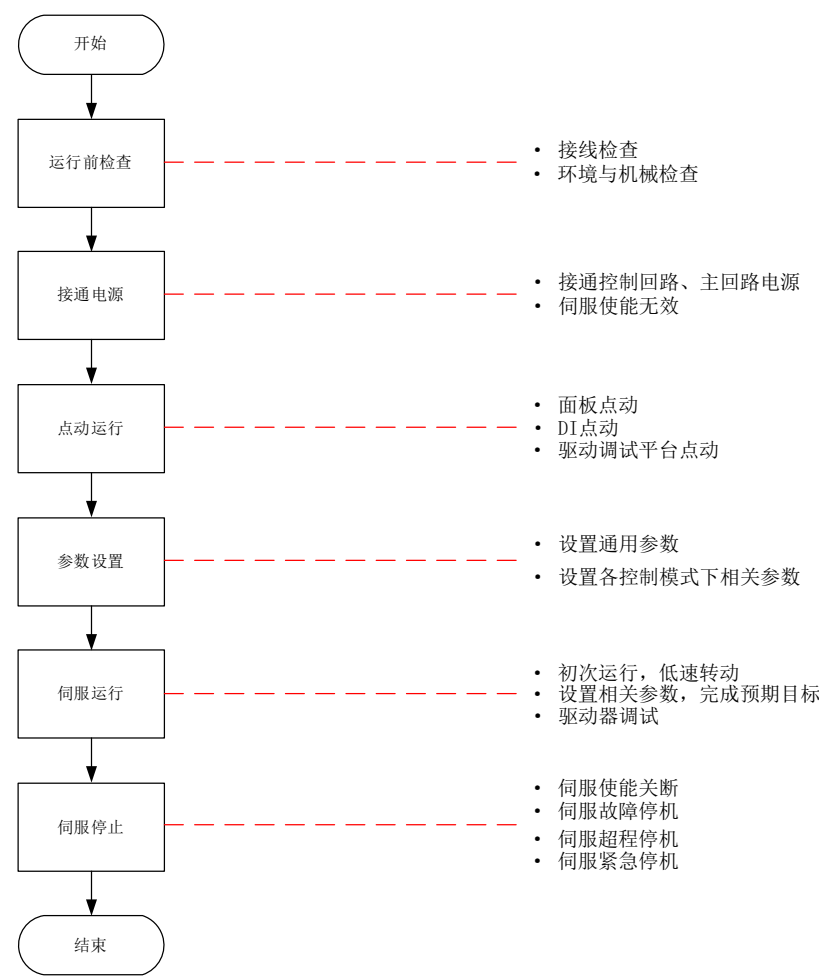
图 6-2 伺服设定流程
