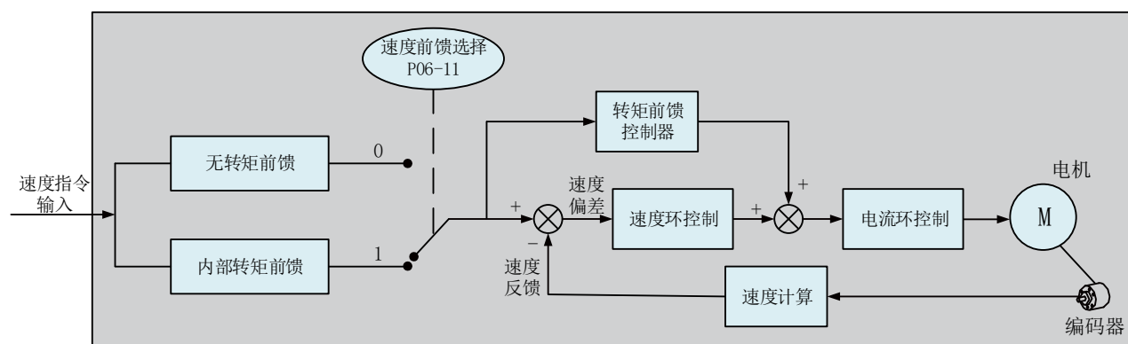
图 7-10 转矩前馈控制操作图
