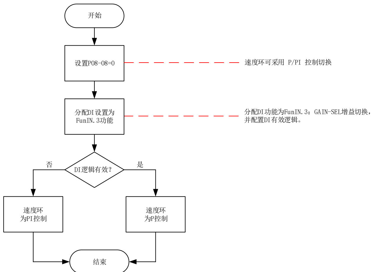
图 7-7 P08-08=0 增益切换流程图
