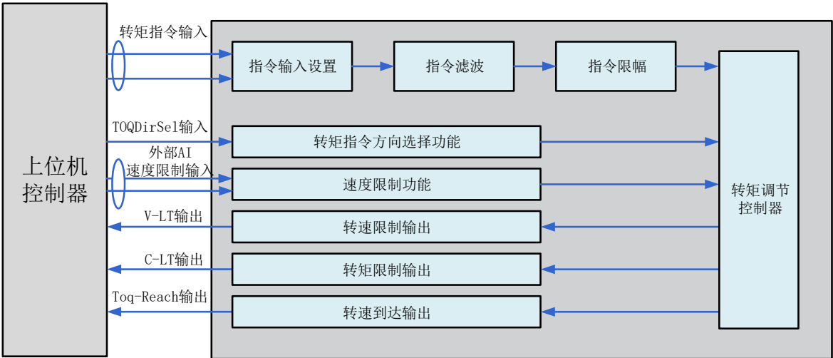
图 6-84 伺服驱动器与上位机信号交互图
