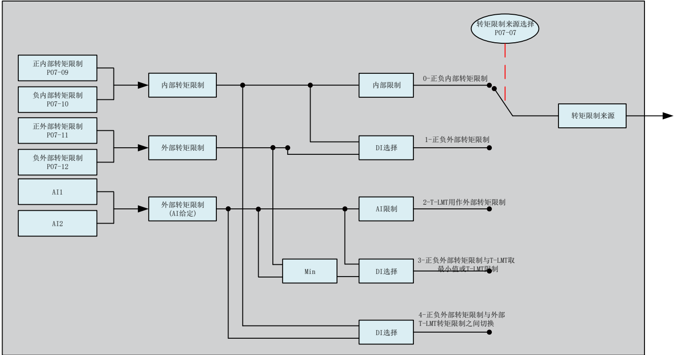
图 6-96 转矩限制来源
