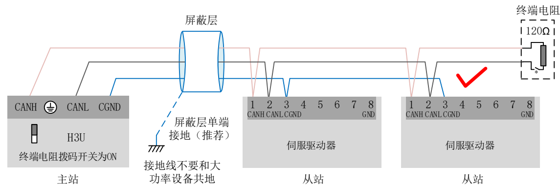
图4-14 正确的CAN连接方法
