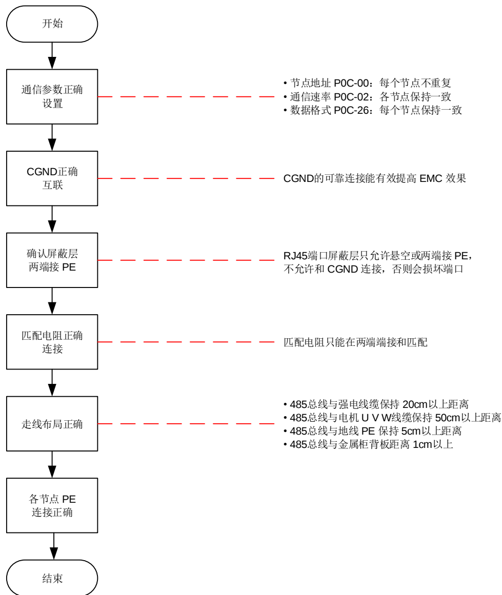
图10-15 485通信现场问题定位流程图
