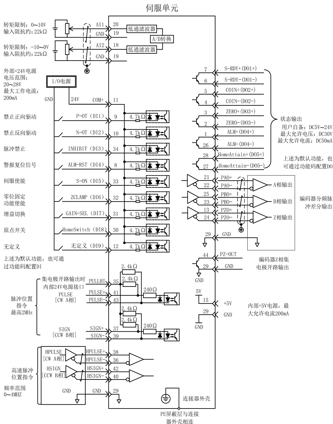
图 4-28 位置模式配线图
