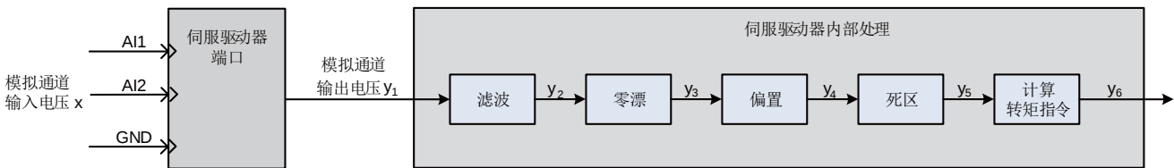
图 6-88 伺服驱动器 AI 处理流程
