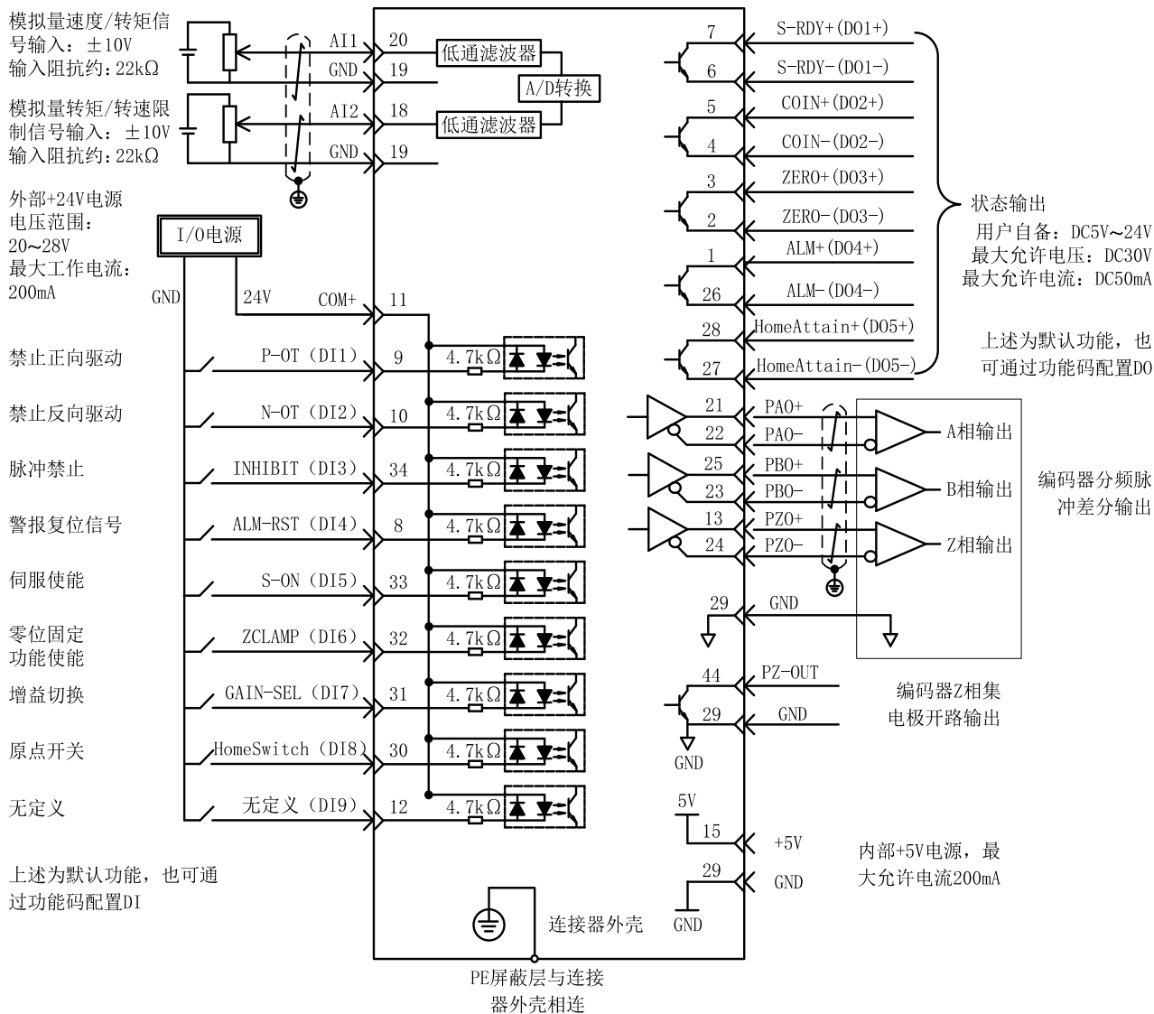
图 4-29 速度模式配线图
