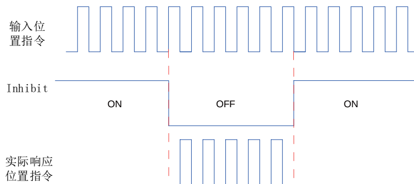
图 6-32 位置指令禁止功能波形举例
