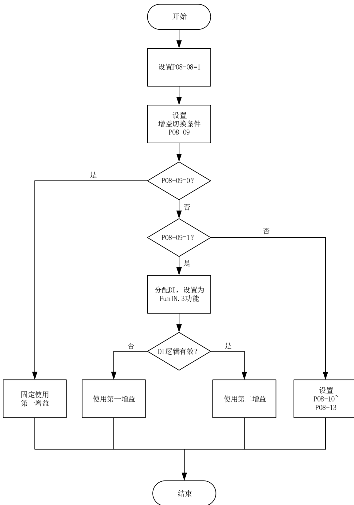
图 7-8 P08-08=1 增益切换流程图
