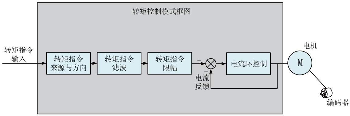
图 6-83 转矩控制框图
