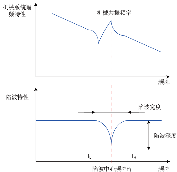
图 7-13 陷波器的抑制原理
