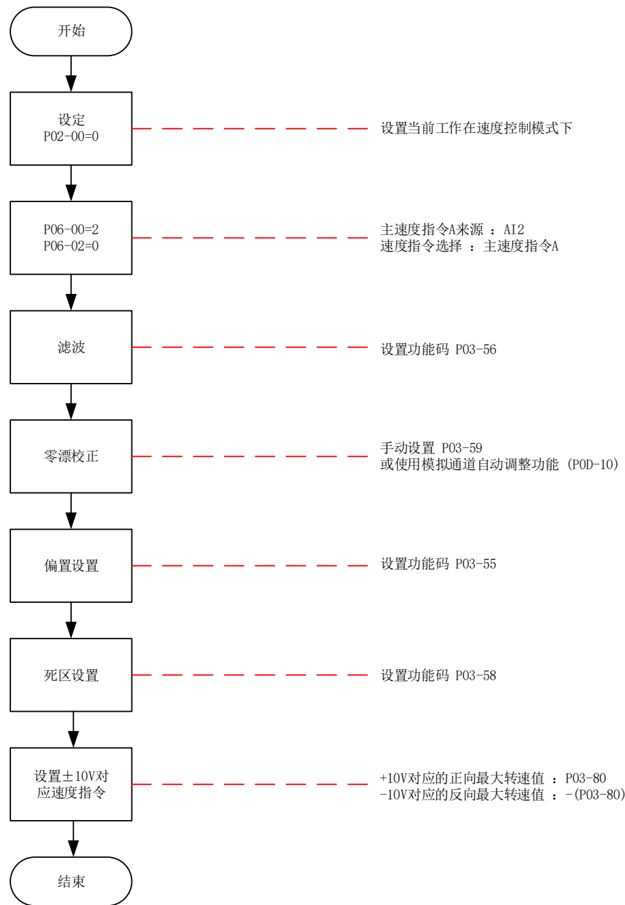
图 6-67 模拟量电压速度指令操作流程图
