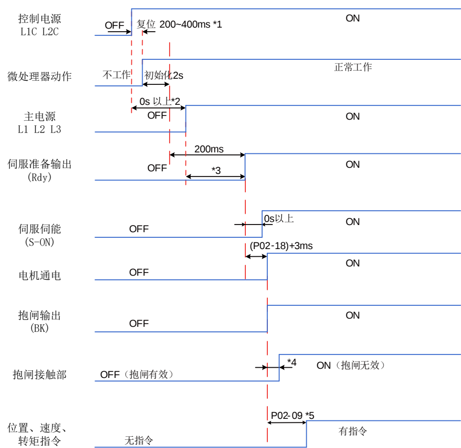
图6-12 电源接通时序图
