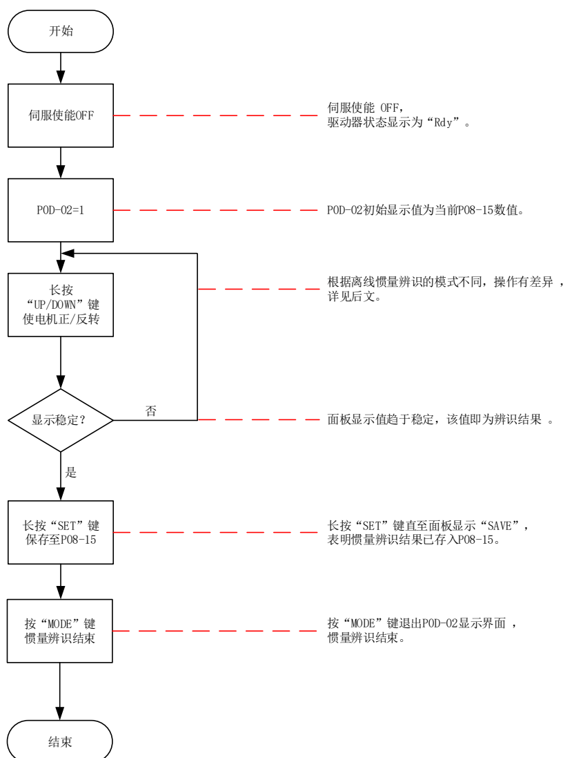
图 7-3 离线惯量辨识流程图
