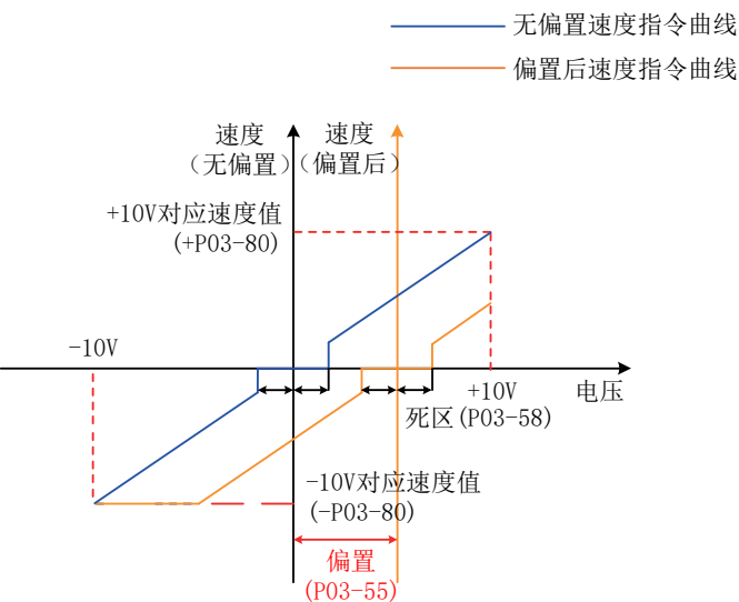
图 6-71 偏置后 AI2 示意图
