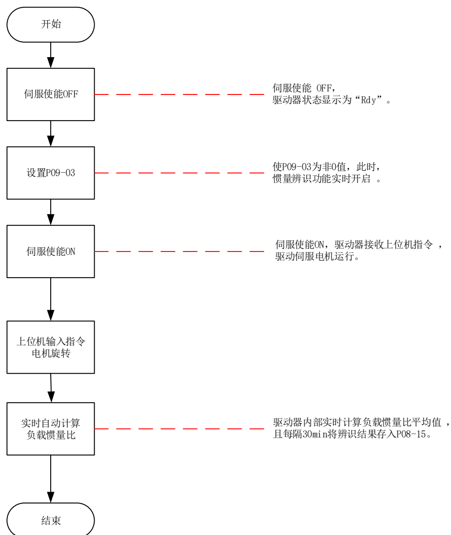
图 7-4 在线惯量辨识操作流程
