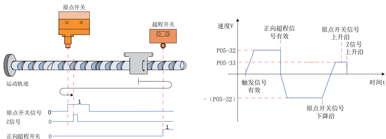
图 6-54 模式 4 原点回零电机运行曲线③与转速说明
