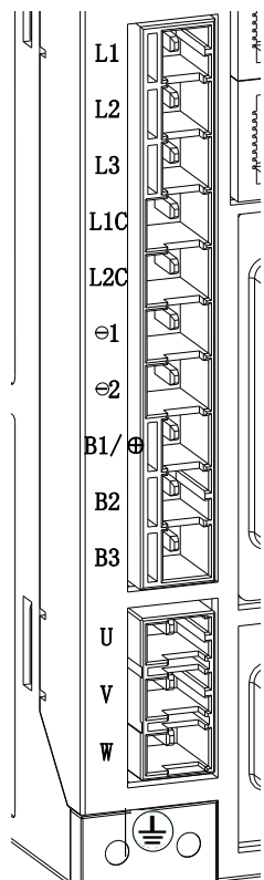
图4-2 伺服驱动器端子排排布
