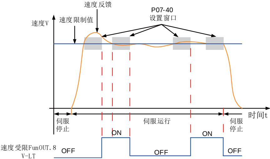
图 6-107 速度限制 D0 输出波形举例
