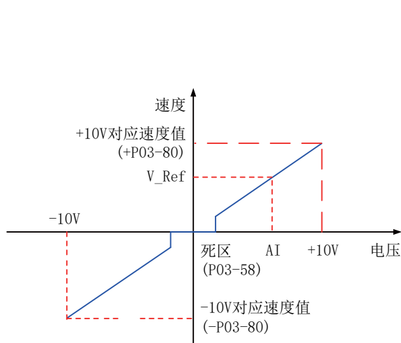
图 6-70 无偏置 AI2 示意图
