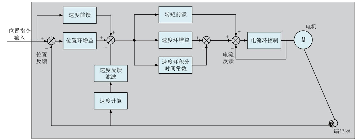
图 7-6 手动增益基本说明框图
