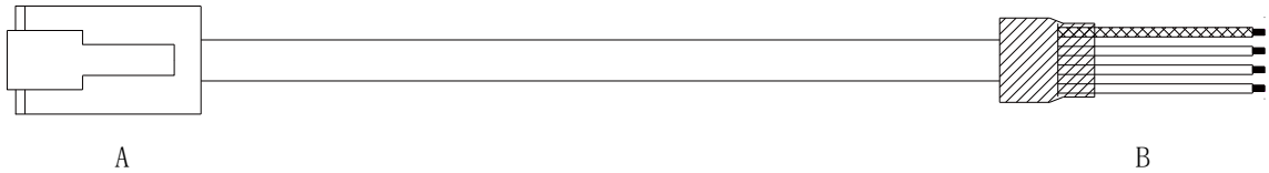
图4-16 PLC和伺服通信线缆外观示例图
