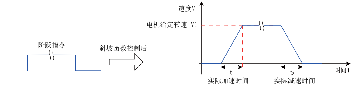
图 6-76 斜坡函数定义示意图
