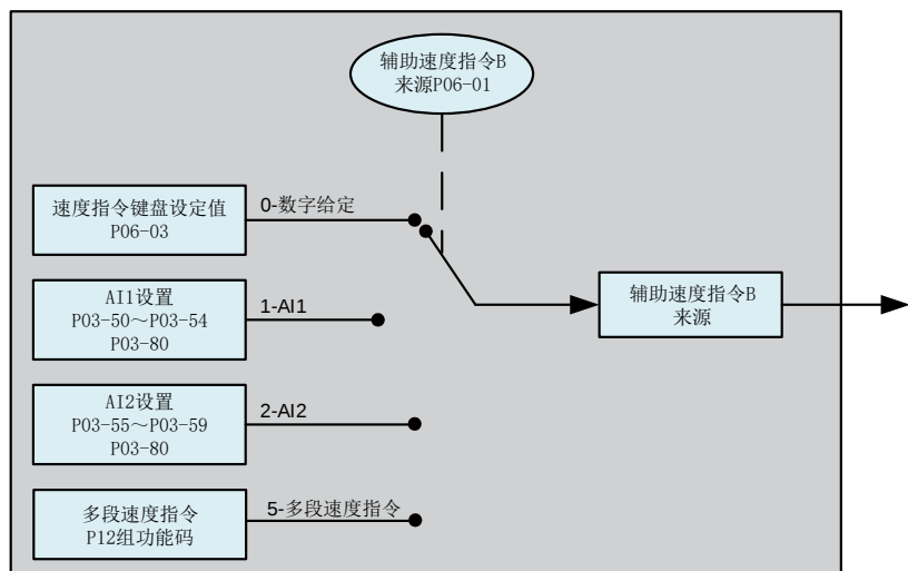
图 6-72 辅助速度指令 B 来源图
