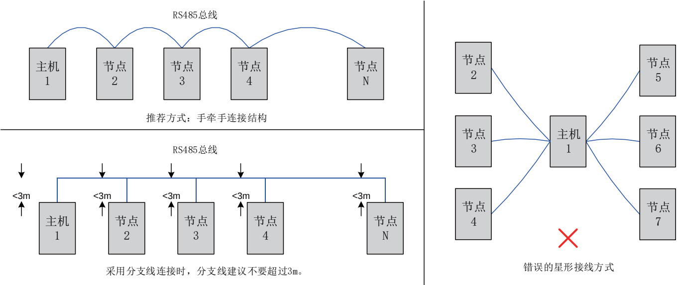
图10-12 三种多节点连接方式示意图
