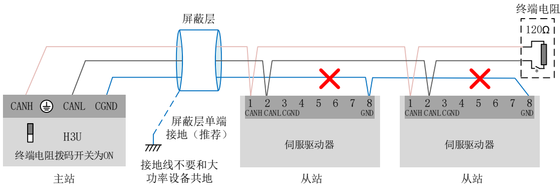
图4-15 错误的CAN连接方法
