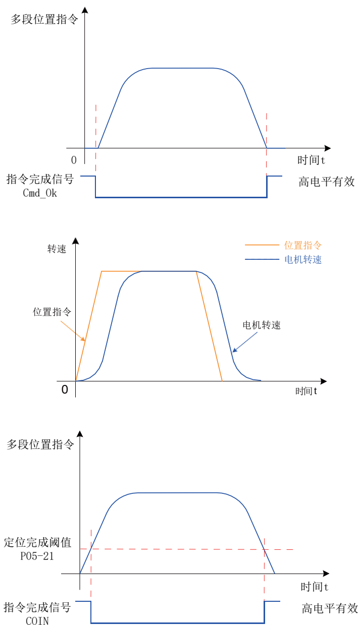
图 6-41 定位完成/接近功能说明
