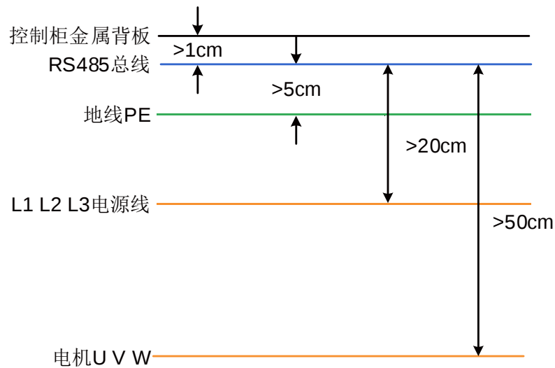
图10-8 线缆布置示意图
