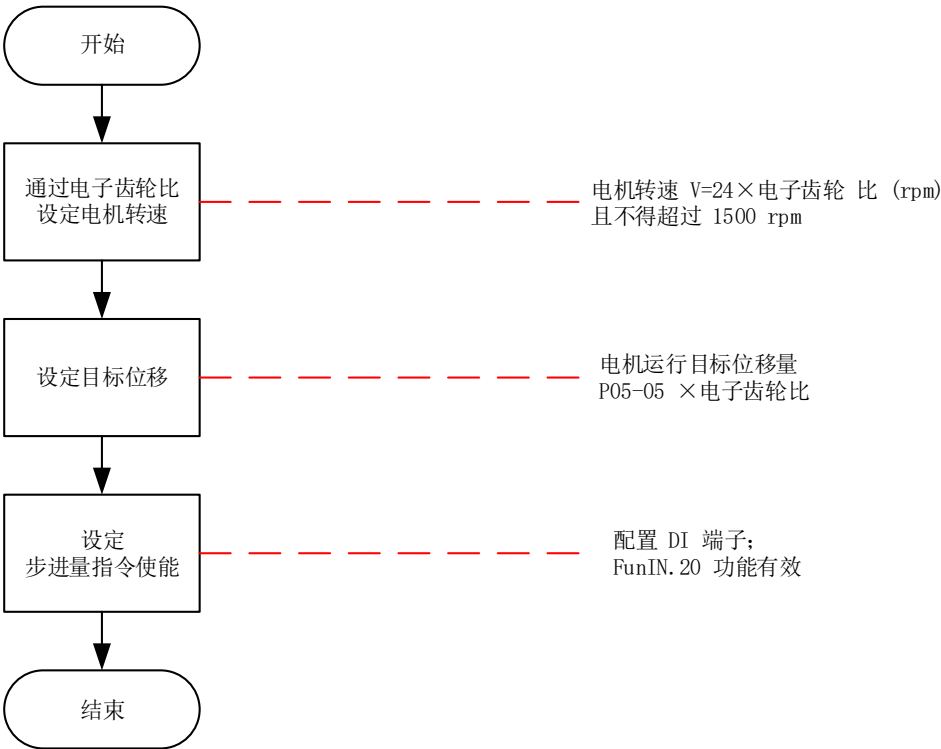
图 6-27 步进量指令来源设置流程
