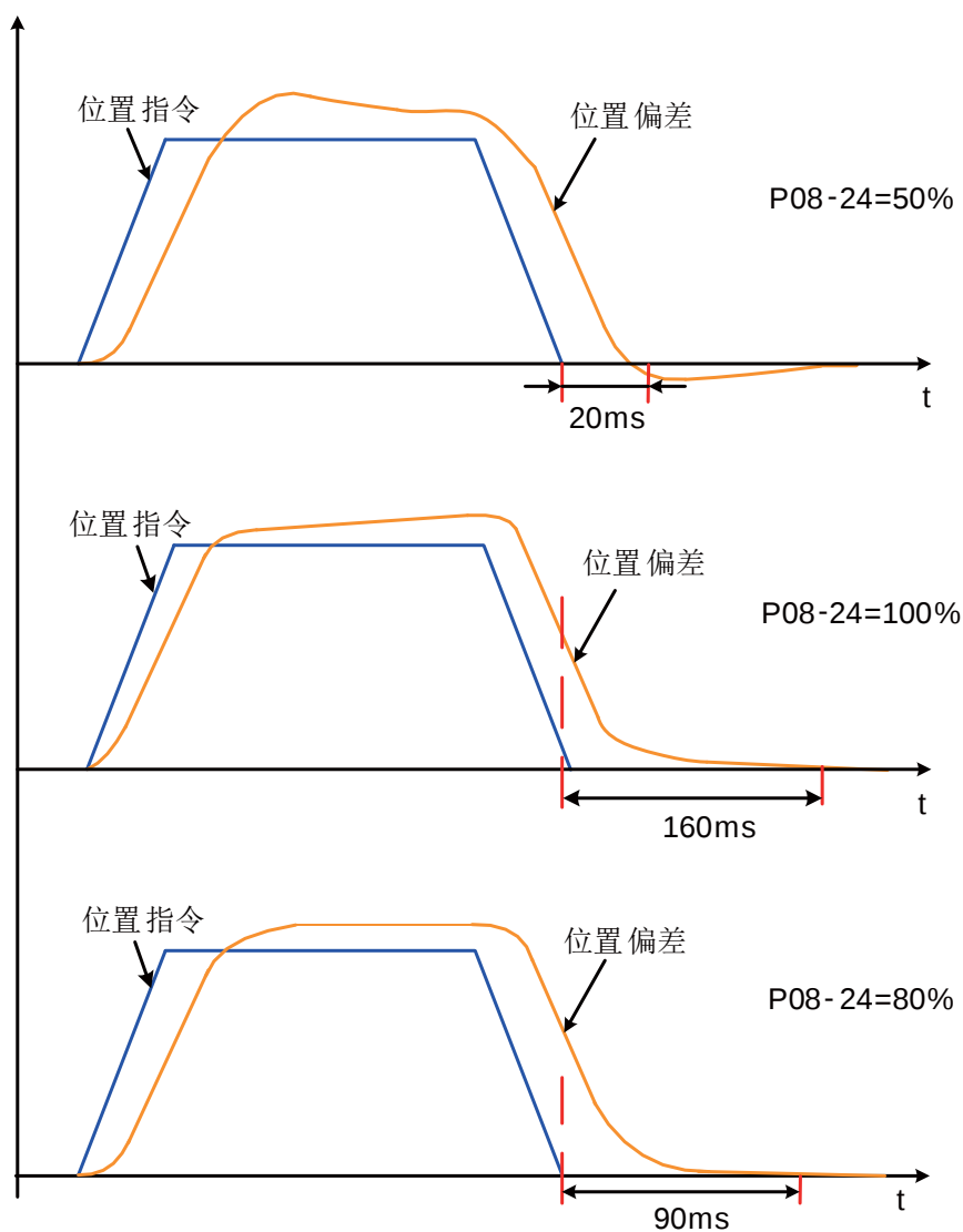
图 7-11 伪微分调节控制举例
