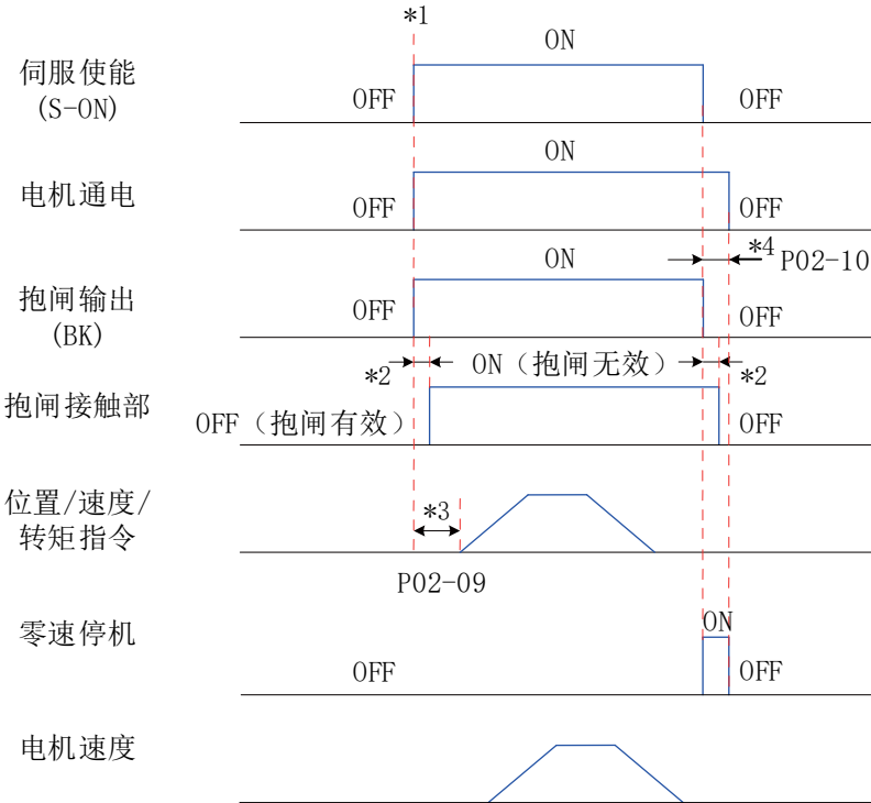
图 6-5 电机静止时抱闸时序图
