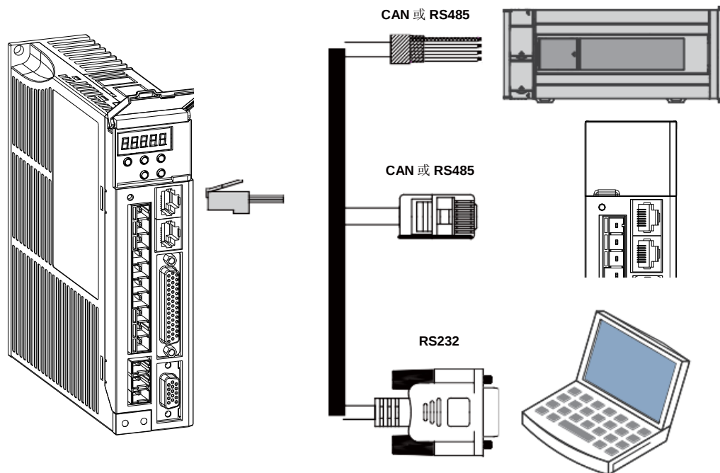
图4-11 通信配线示意图
