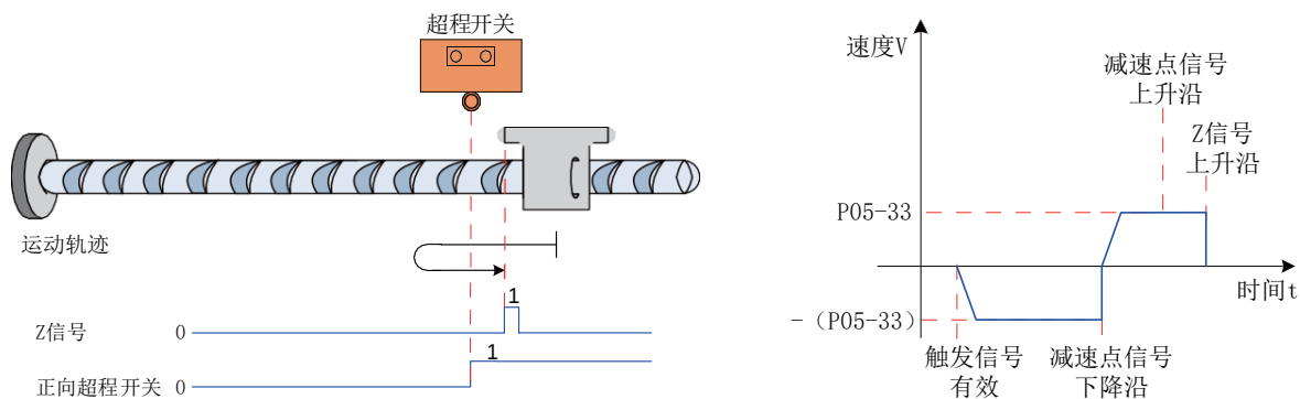
图 6-58 模式 8 原点回零电机运行曲线②与转速说明
