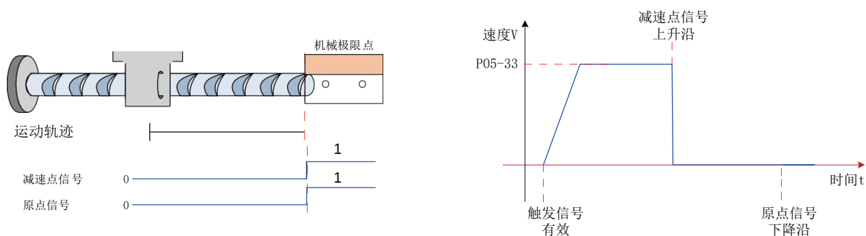
图 6-59 模式 10 原点回零电机运行曲线与转速说明
