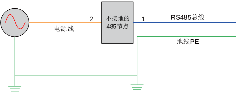
图10-13 抑制外部干扰示意图
