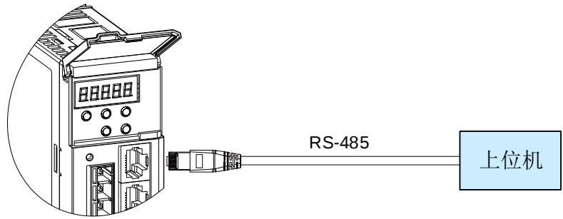
图10-2 RS-485连接示意图
