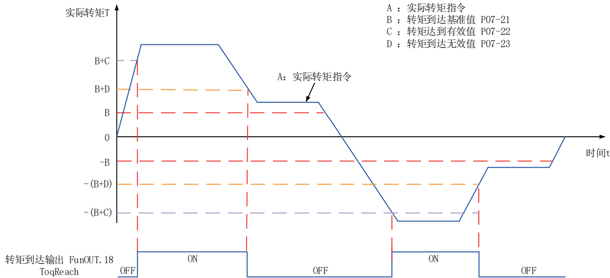
图 6-108 转矩到达输出波形举例
