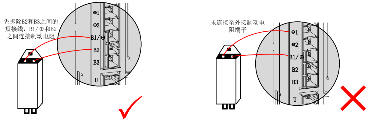
图4-3 外接制动电阻的连接示意图
