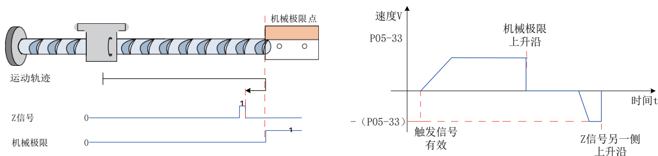
图 6-60 模式 12 原点回零电机运行曲线与转速说明
