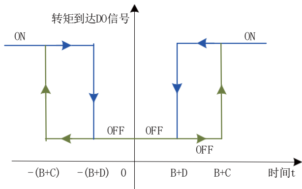
图 6-109 转矩到达输出有效说明
