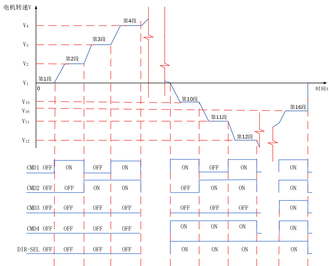
图 6-74 多段速度曲线举例
