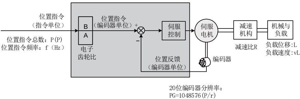
图 6-36 位置指令(指令单位)、负载位移与电子齿轮比之间的关系
