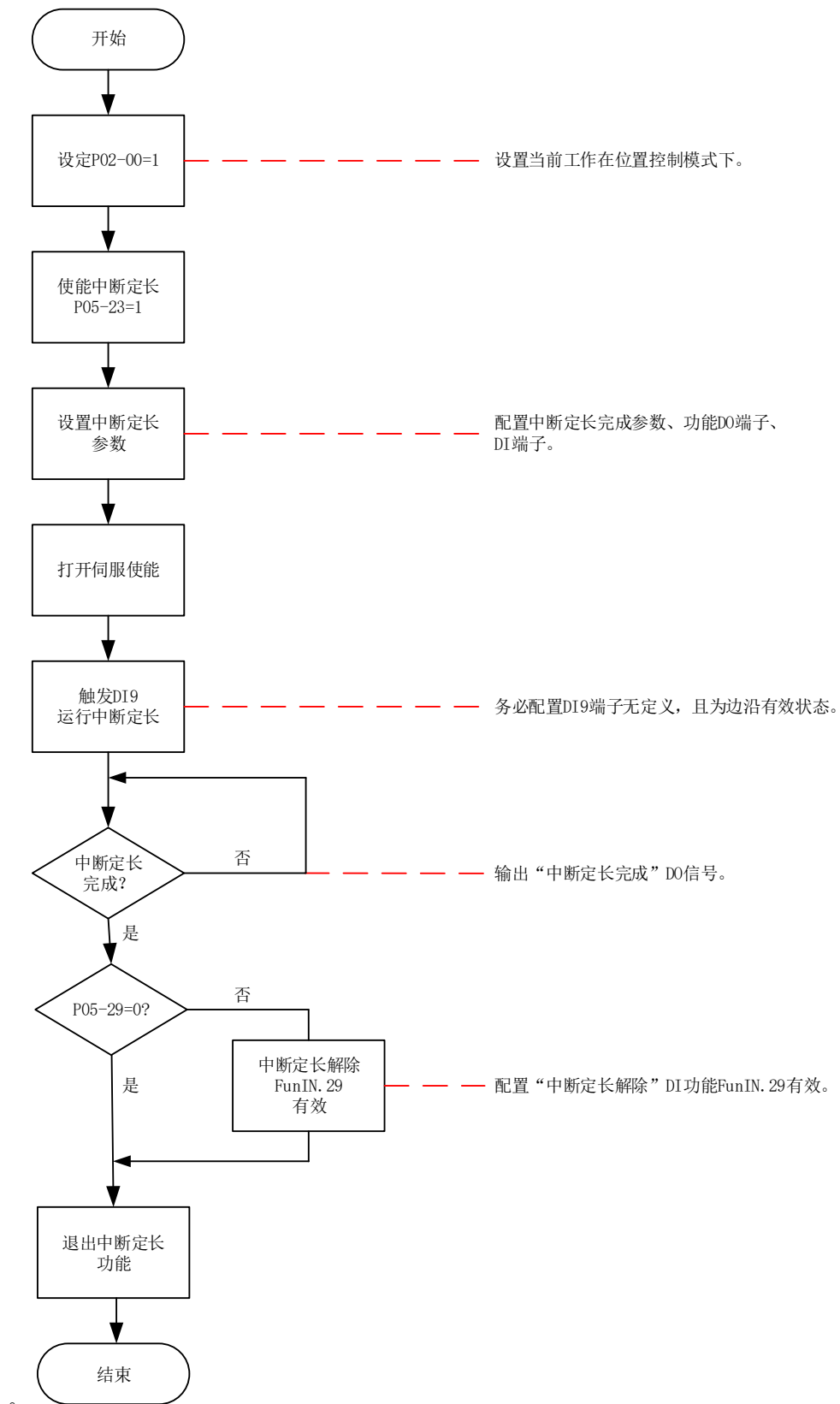
图 6-44 中断定长功能信号流程图
