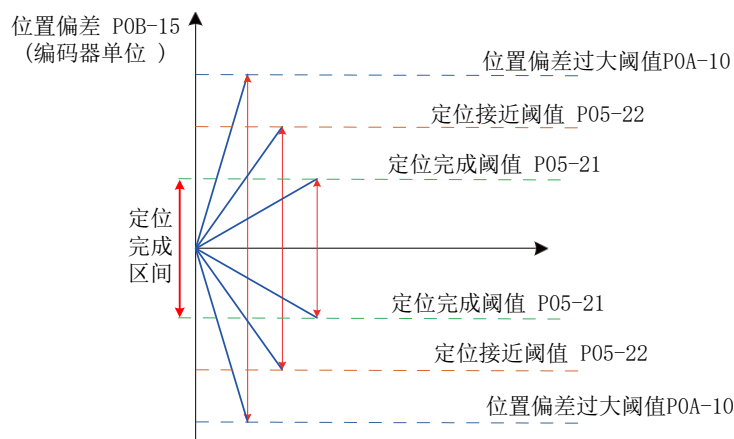
图 6-42 位置偏差相关信号
