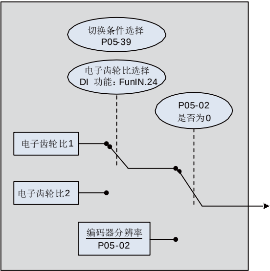
图 6-35 电子齿轮比设定操作流程
