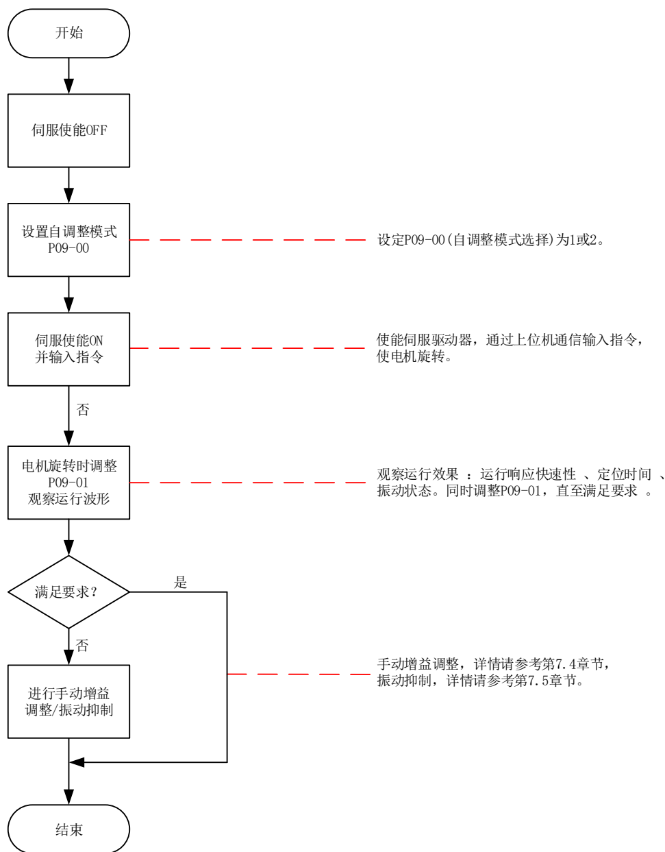
图 7-5 自动增益调整步骤
