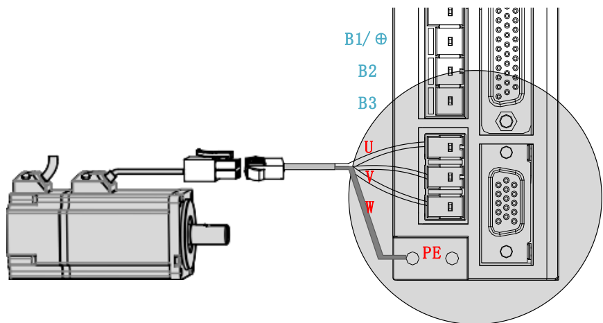
图4-6 伺服驱动器输出与伺服电机连接举例
