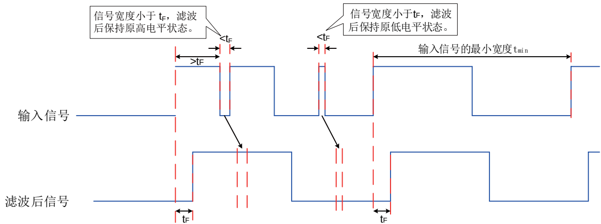
图 6-26 滤波信号波形举例
