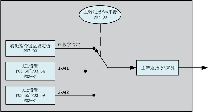
图 6-86 主转矩指令 A 来源说明
