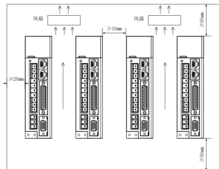
图3-1 伺服驱动器安装示意图
