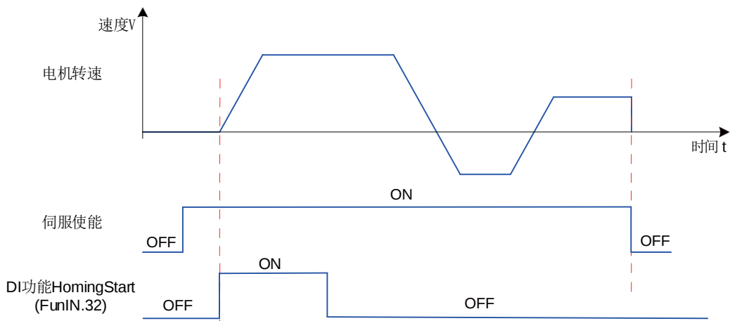
图 6-62 时序图举例
