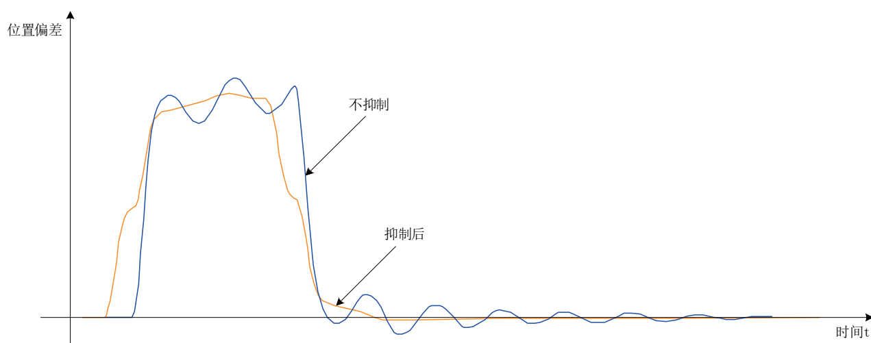
图 7-18 低频共振抑制效果图
