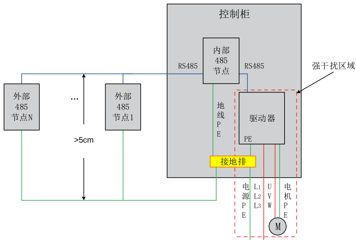
图10-6 区域布置示意图
