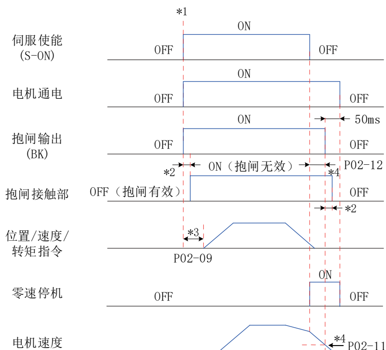
图 6-6 电机旋转时抱闸时序图
