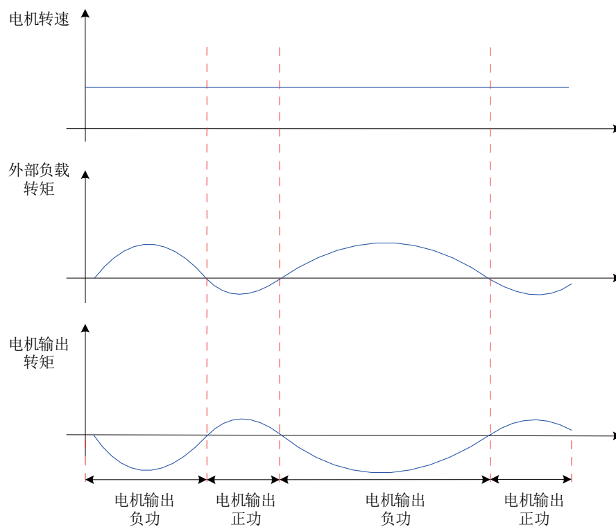
图6-11 外部负载扭矩存在情况下曲线举例
