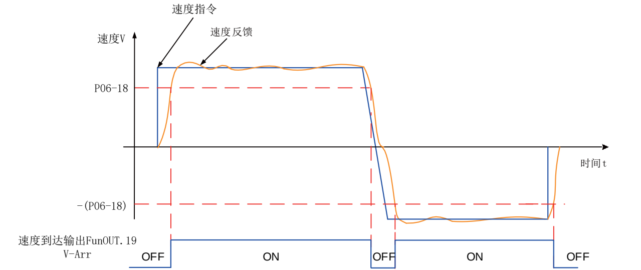
图 6-81 速度到达信号波形图
