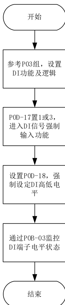
图 5-8 DI 信号强制输入设定步骤示意图
