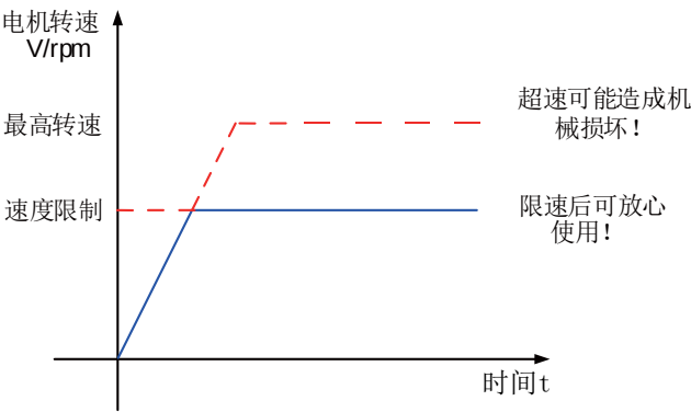
图 6-103 转矩模式速度限制示意图
