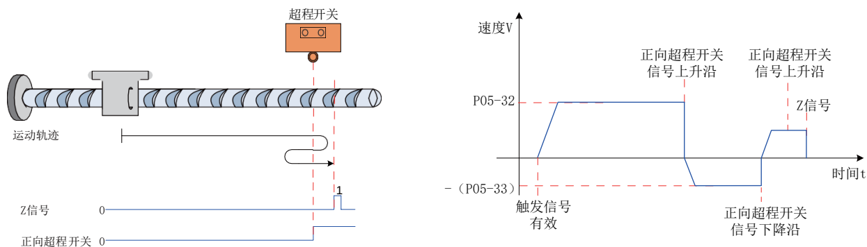
图 6-57 模式 8 原点回零电机运行曲线①与转速说明
