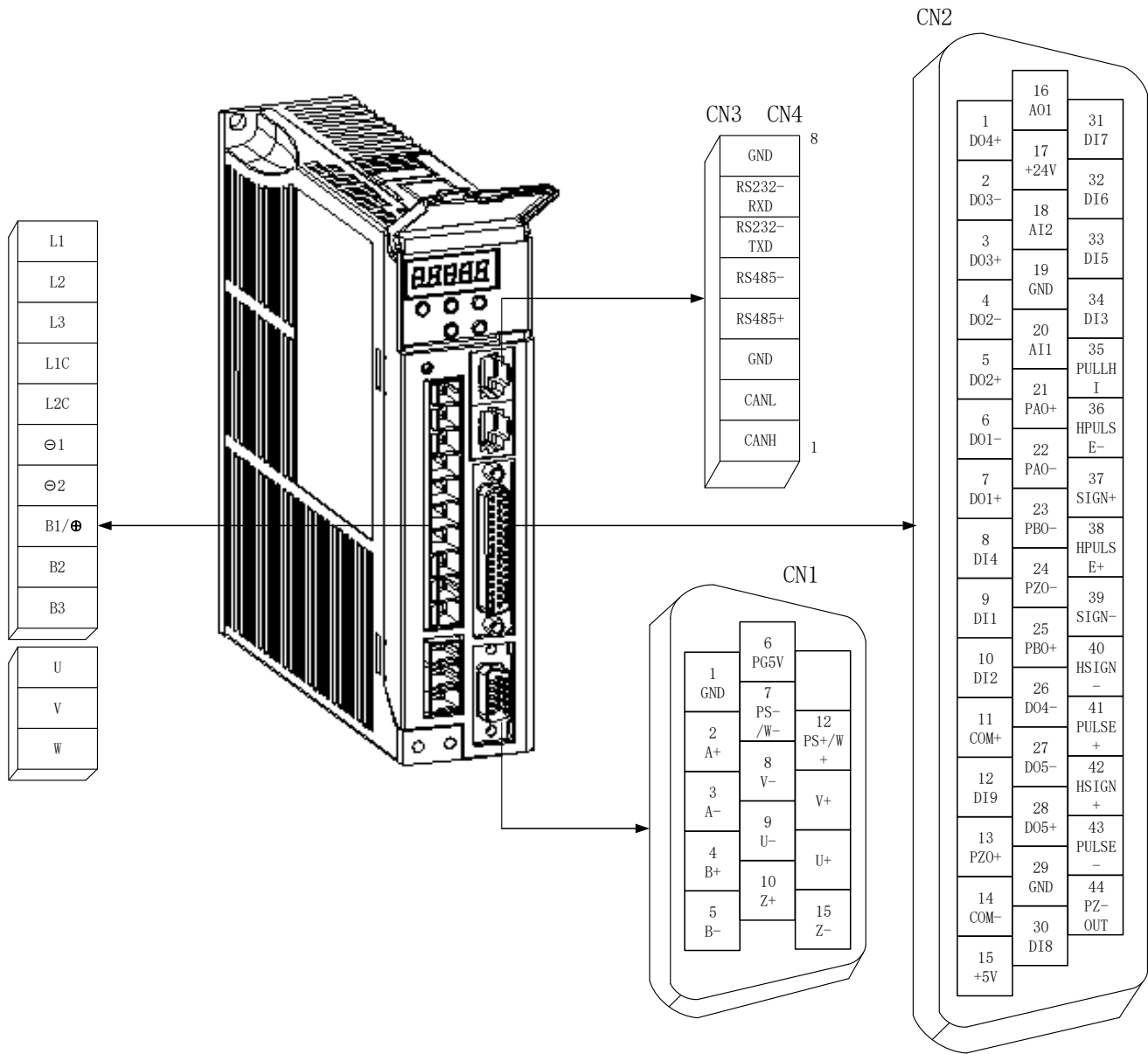
图4-1 伺服驱动器端子引脚分布图
