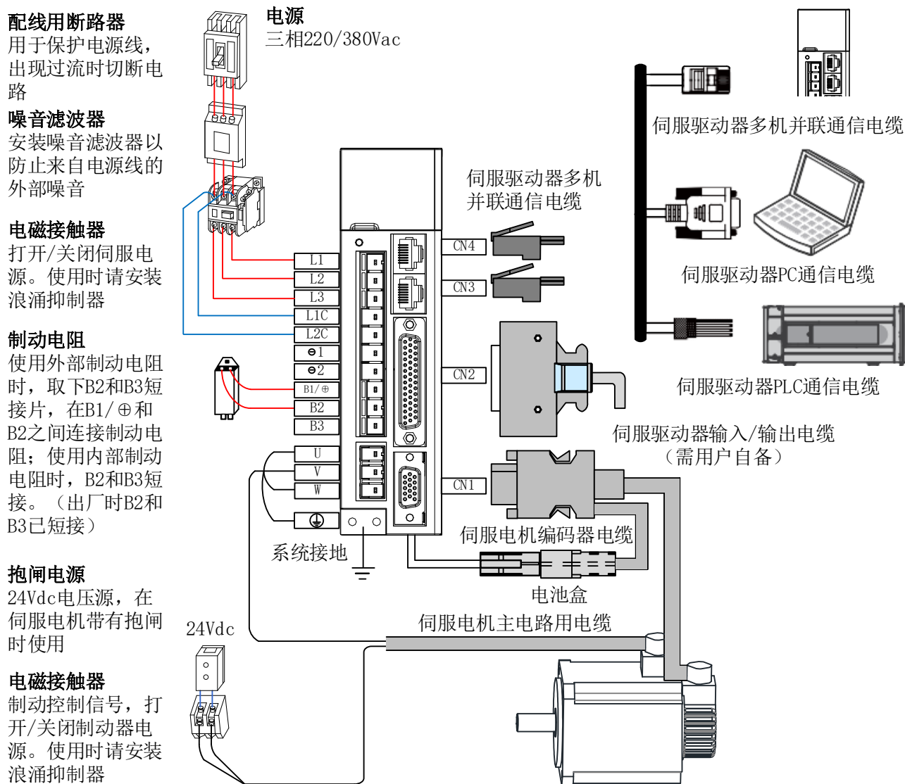
图2-3 系统配线图举例
