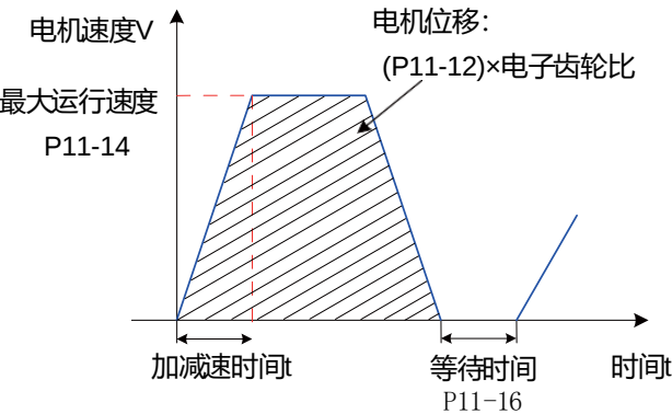
图 6-31 第 1 段电机运行曲线
