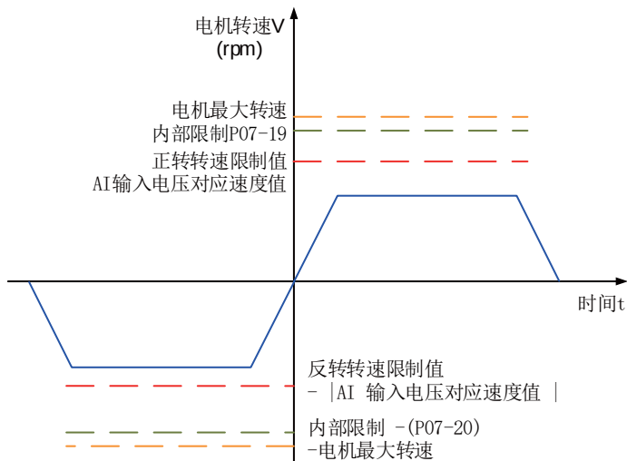
图 6-106 P07-17=1 速度限制曲线图
