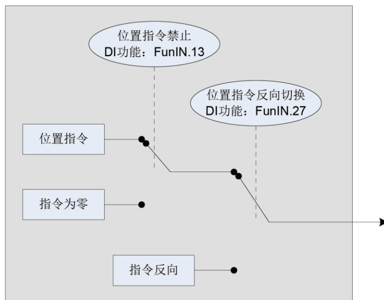
图 6-23 位置指令输入设置框图
