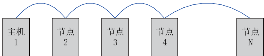
图10-3 推荐手牵手连接结构示意图
