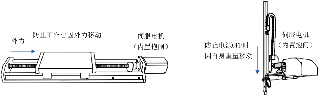
图 6-3 抱闸应用示意图
