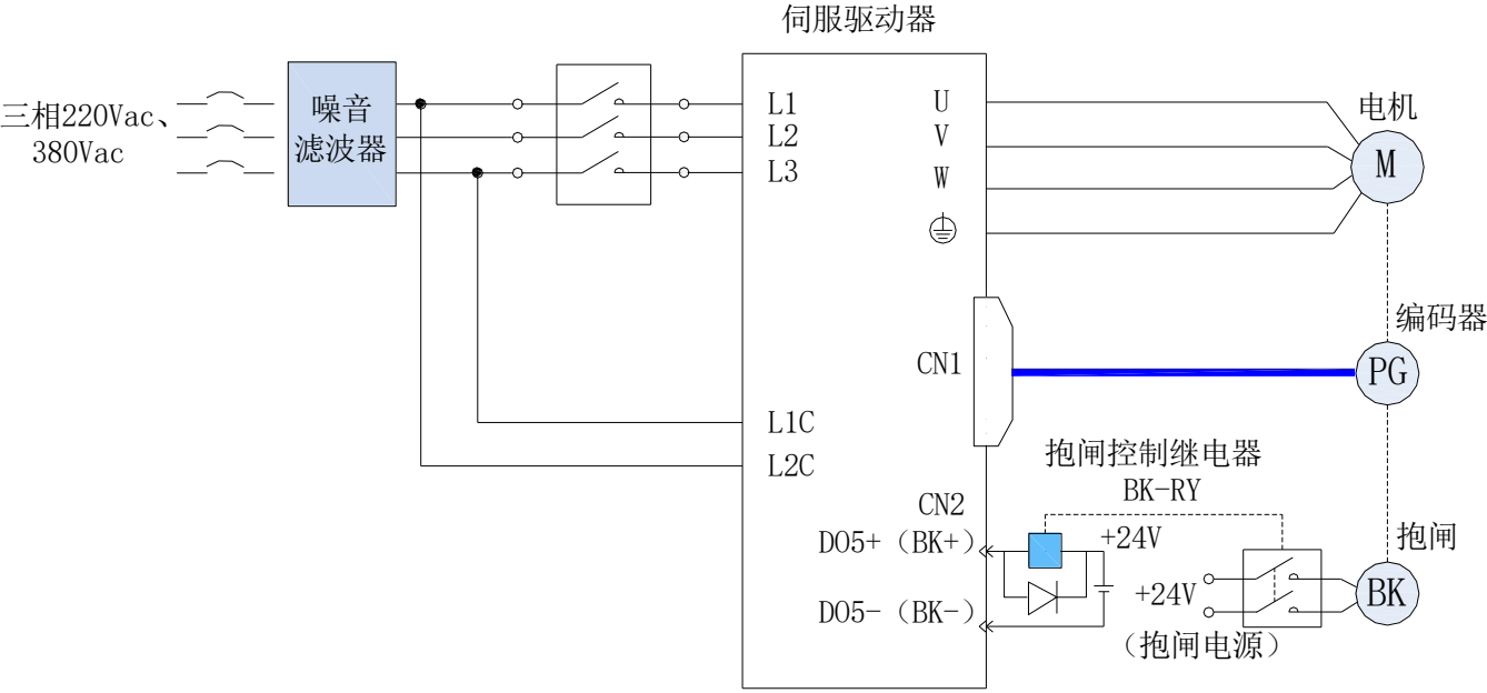
图 6-4 抱闸配线图
