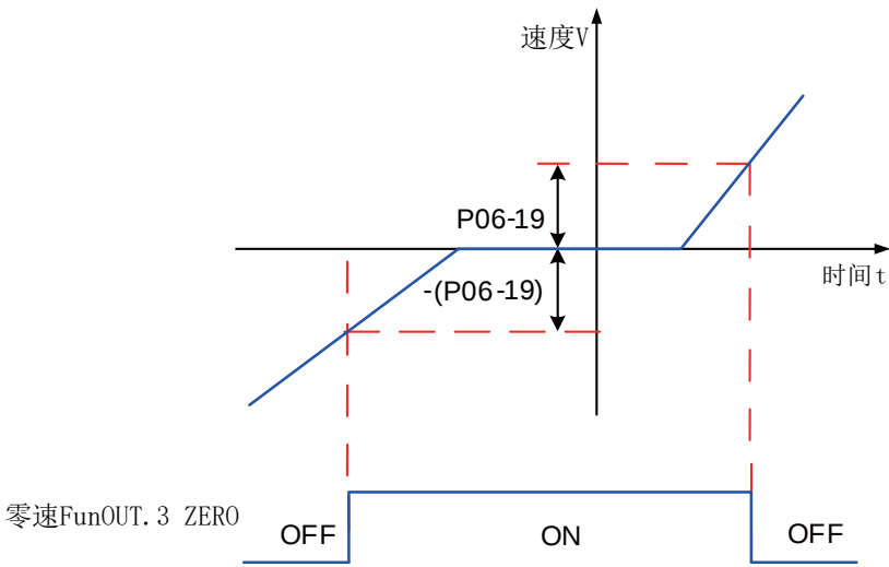
图 6-82 零速信号波形图
