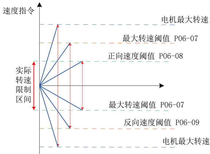
图 6-78 速度指令限幅举例说明
