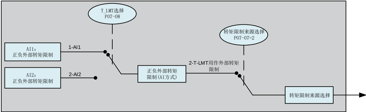
图 6-99 P07-07=2 转矩限制来源
