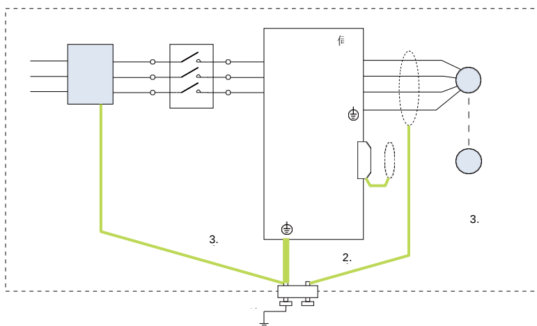
图4-22 抗干扰配线实例
