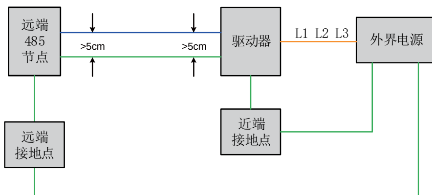
图10-7 地线PE配线示意图
