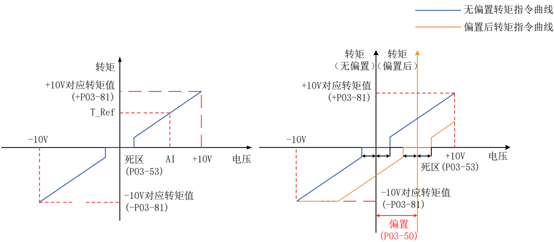
图 6-90 无偏置 AI2 示意图图 6-91 偏置后 AI2 示意图
