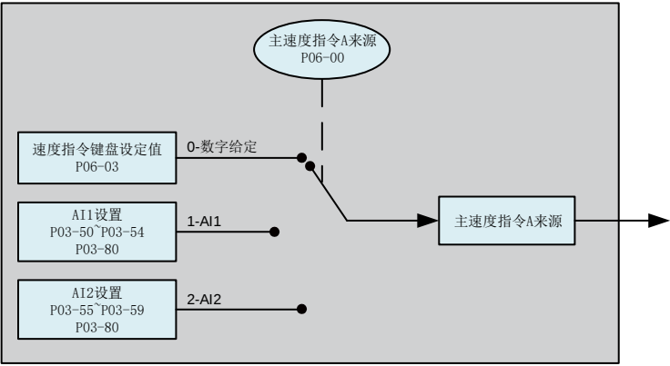
图6-66 主速度指令A来源图
