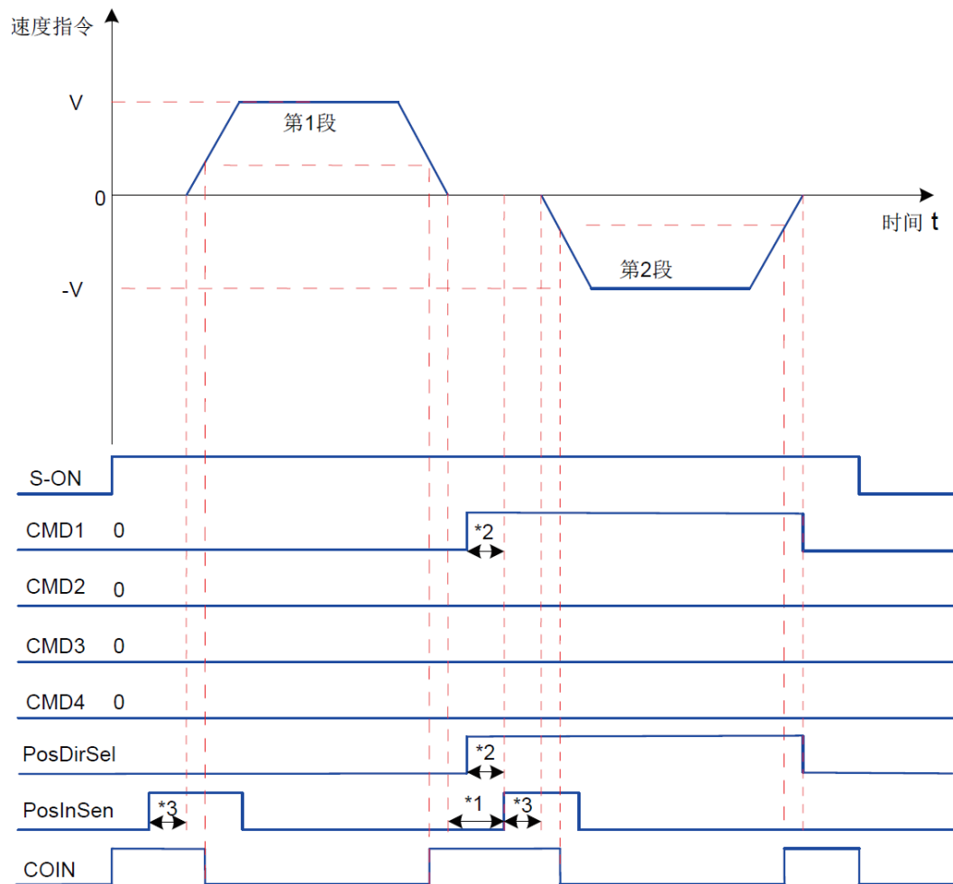
图 6-30 多段位置时序图
