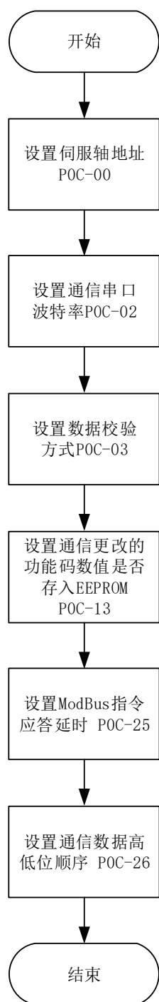
图10-9 通信参数设定流程
