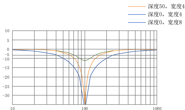
图 7-15 陷波器频率特性
