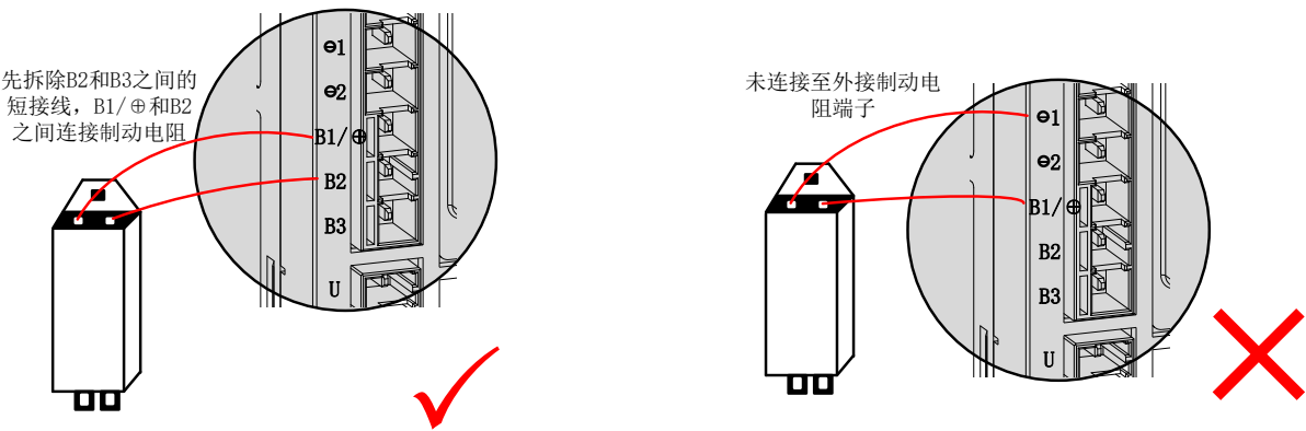
图6-9 外接制动电阻连接示意图
