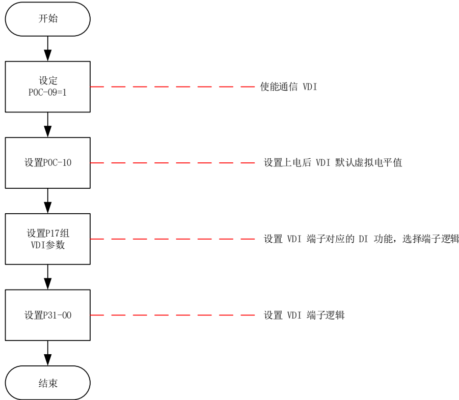
图10-16 VDI使用流程图
