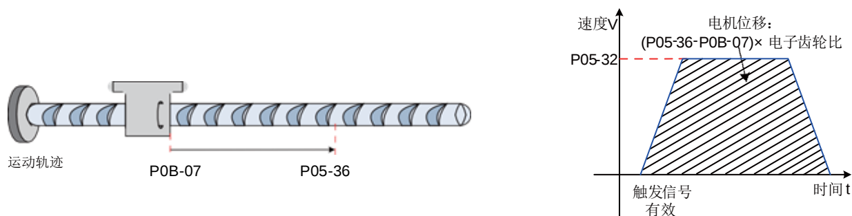
图 6-61 电气回零电机运行曲线与转速说明
