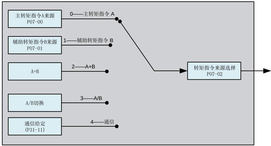
图 6-85 转矩指令来源图
