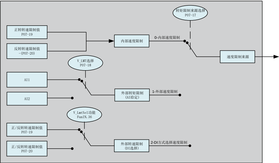
图 6-104 速度限制来源
