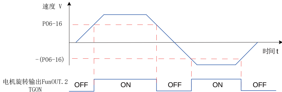
图 6-79 电机旋转信号波形图
