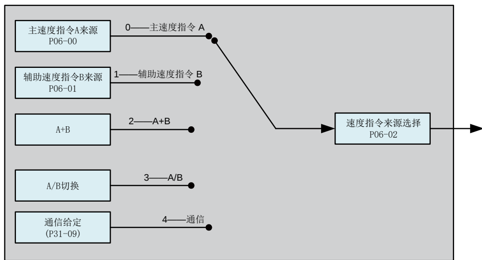
图6-65 速度指令来源图
