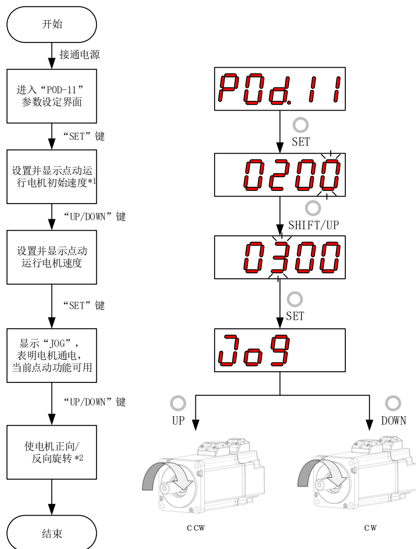
图 5-7 点动运行设定步骤示意图
