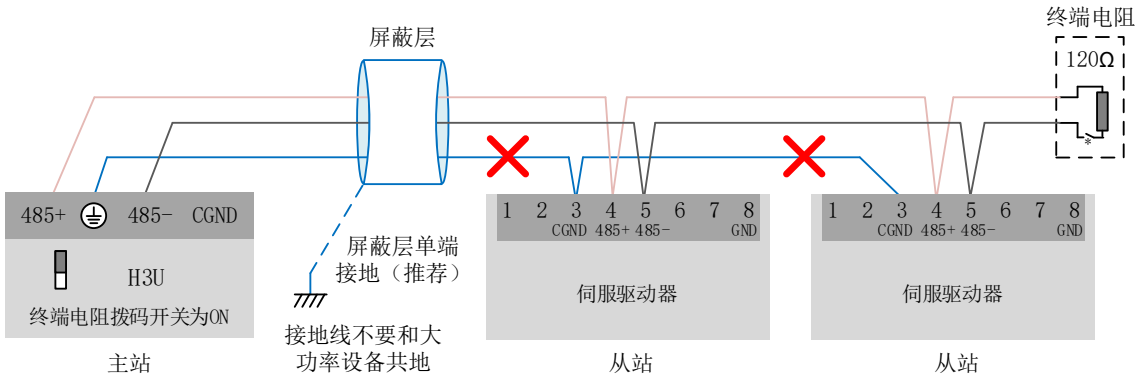
图4-19 错误的485连接方法
