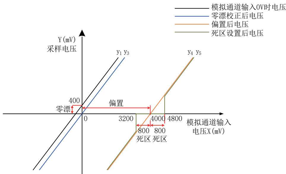
图 6-89 伺服驱动器 AI 处理对应采样电压举例
