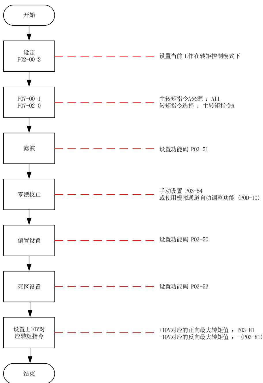
图 6-87 模拟量电压转矩指令操作流程
