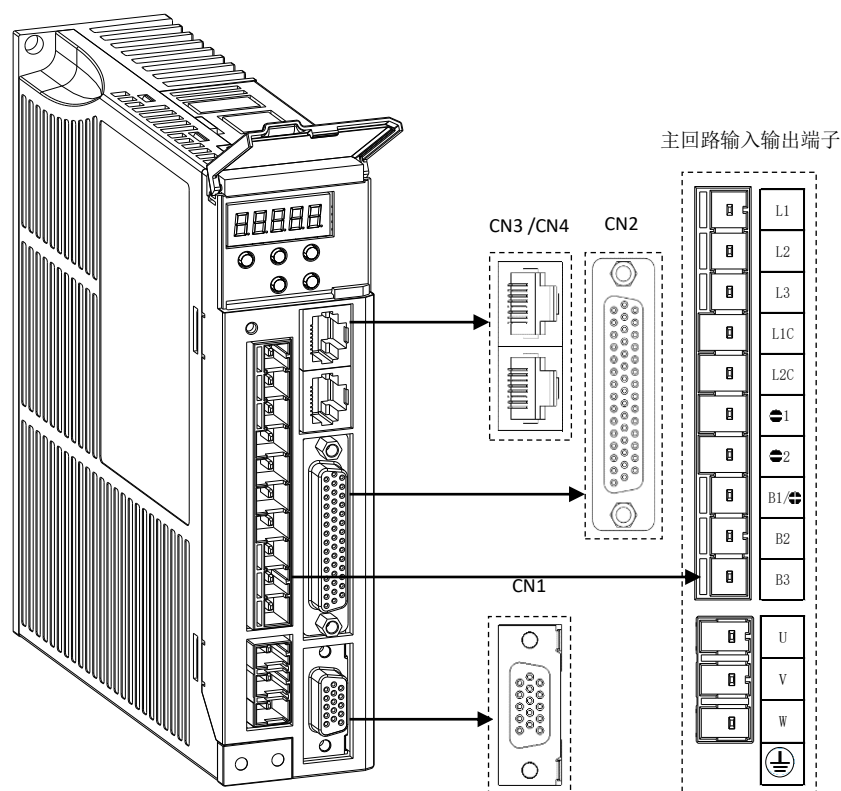
图2-2 伺服驱动器组成
