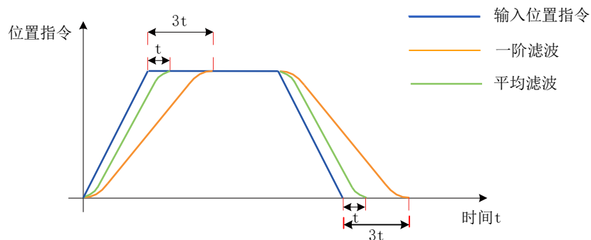
图6-39 梯形位置指令一阶滤波与平均滤波示意图
