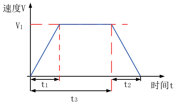
图 6-75 多段速度曲线举例
