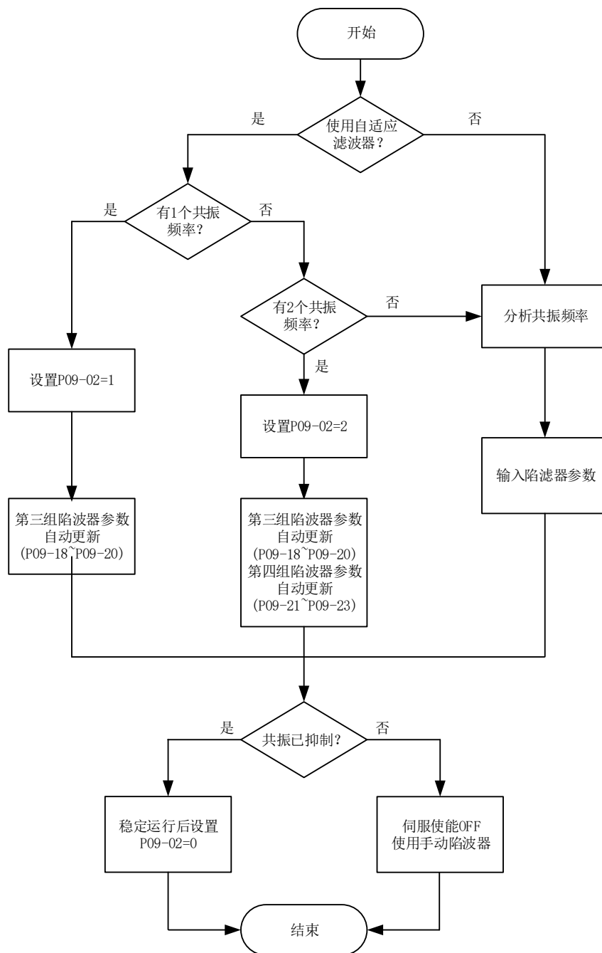
图 7-14 陷波器使用步骤
