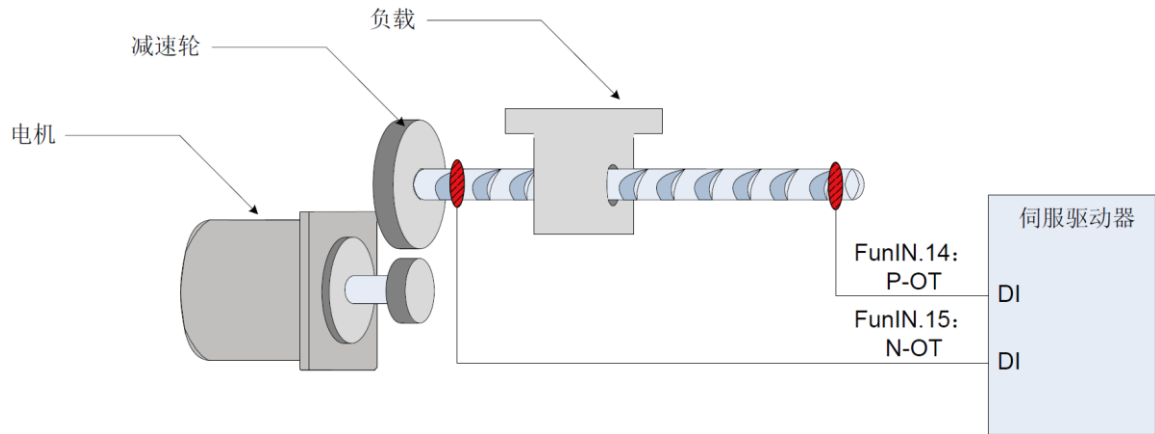
图6-20 限位开关的安装示意图
