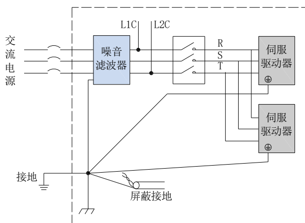
图 4-26 噪音滤波器地线处理示意图
