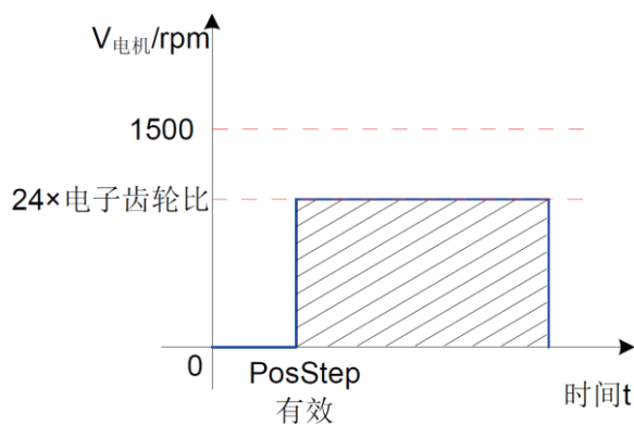
图 6-28 P05-00=1 时，电机运行曲线
