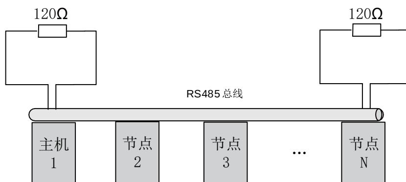
图10-10 终端电阻接入方式示意图
