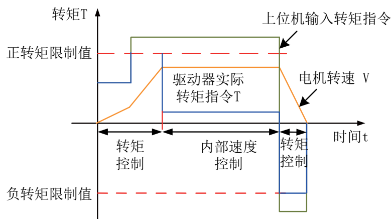
图 6-94 转矩给定与转矩限制
