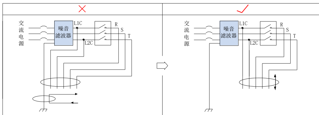
图4-24 噪音滤波器地线与输出配线分离走线示意图
