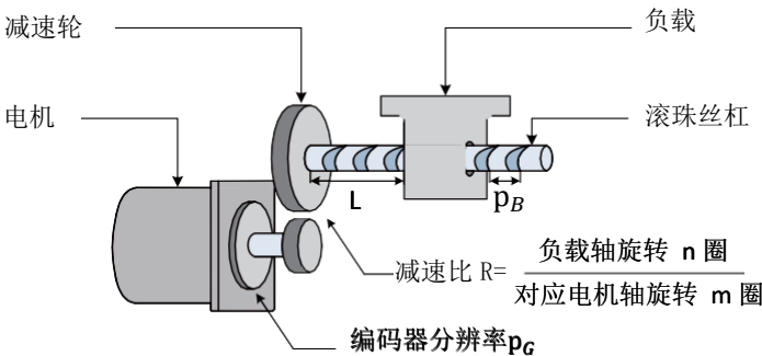
图 6-37 滚珠丝杠图示
