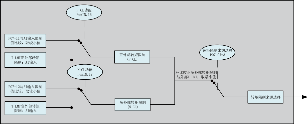
图 6-101 P07-07=3 转矩限制来源
