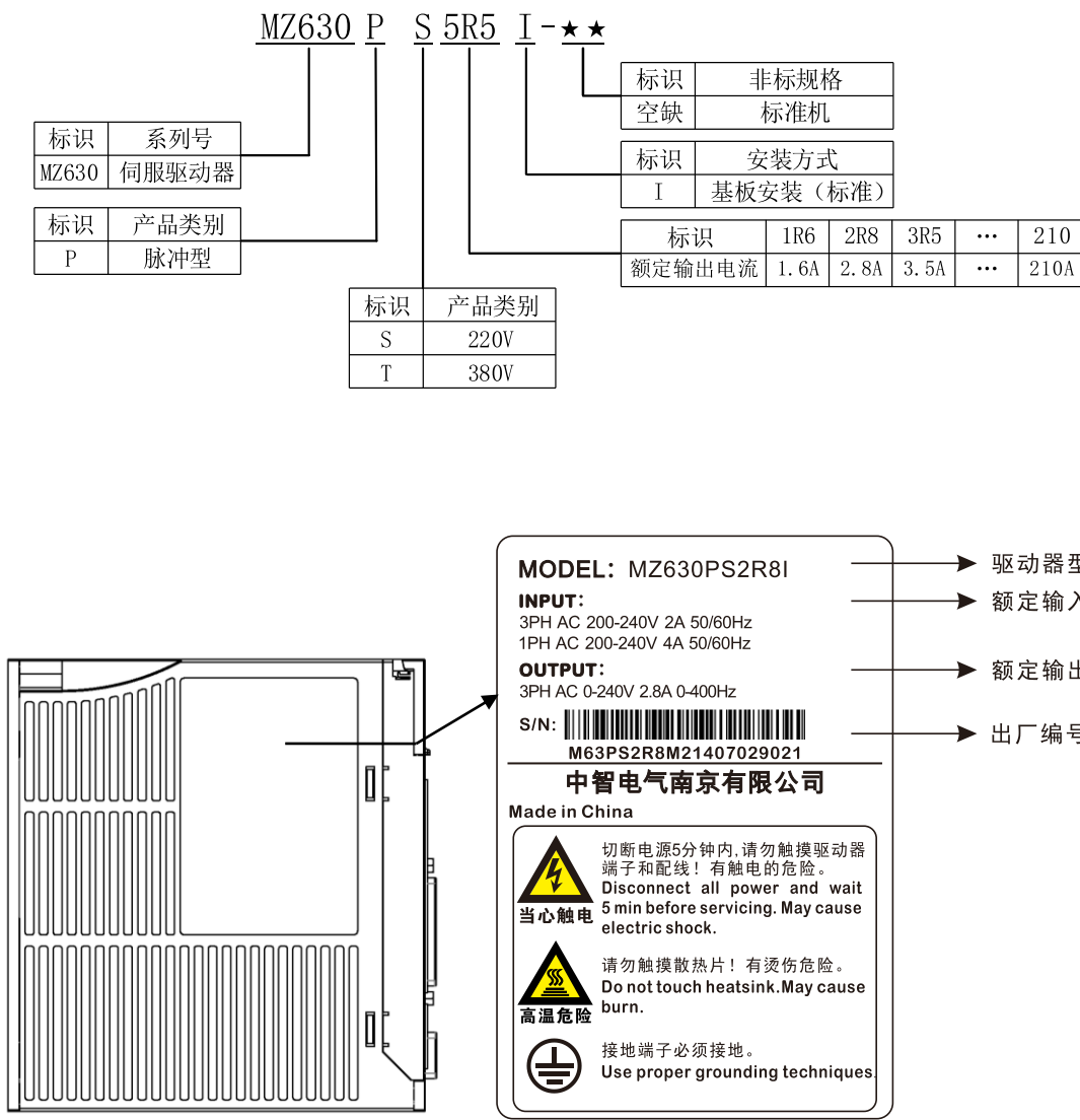
图2-1 驱动器命名与规则
