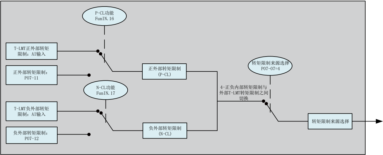
图 6-102 P07-07=4 转矩限制来源
