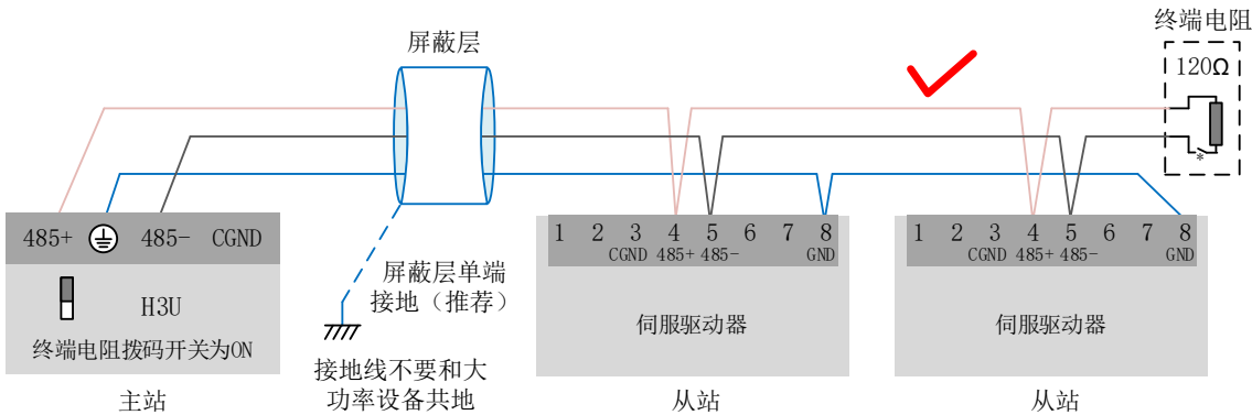
图4-18 正确的485连接方法
