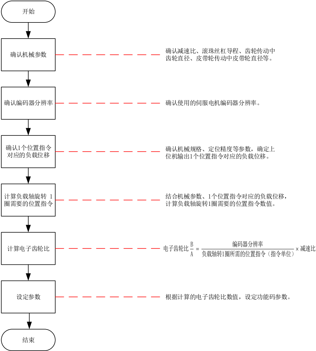
图 6-34 电子齿轮比设定步骤
