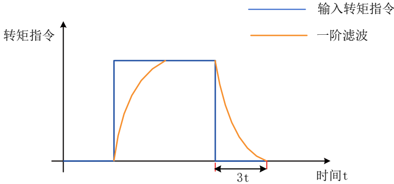
图 6-92 矩形转矩指令一阶滤波示意图
