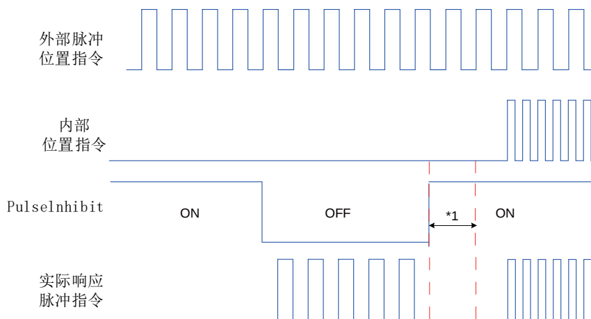
图 6-33 脉冲指令禁止功能波形举例
