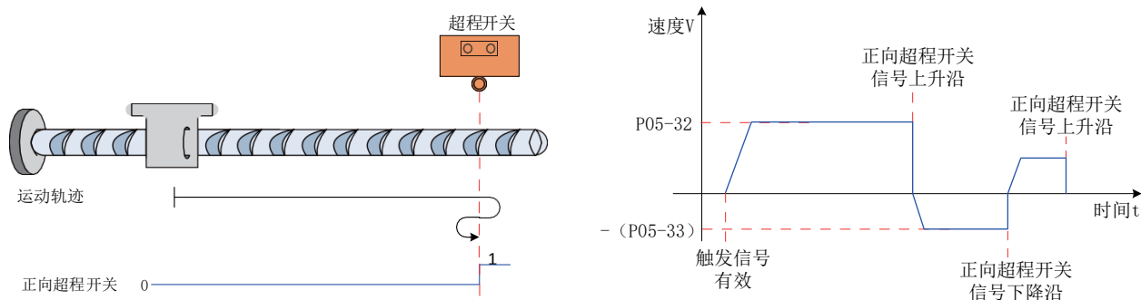
图 6-55 模式 6 原点回零电机运行曲线①与转速说明
