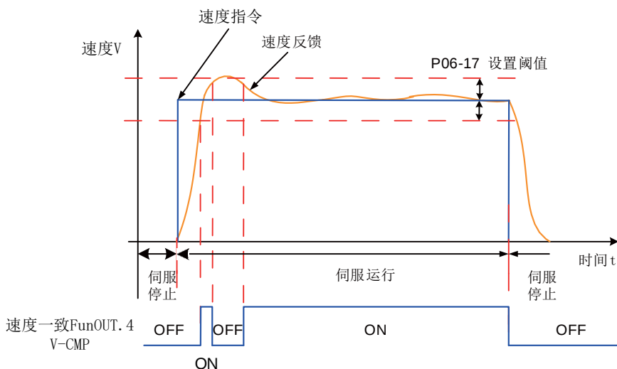
图 6-80 速度一致信号波形图
