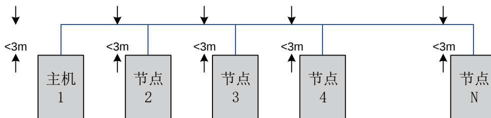
图10-4 分支线连接结构示意图
