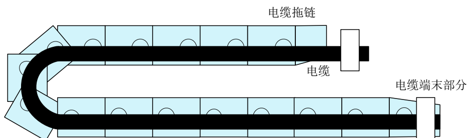
图 4-27 线缆保护链示意图
