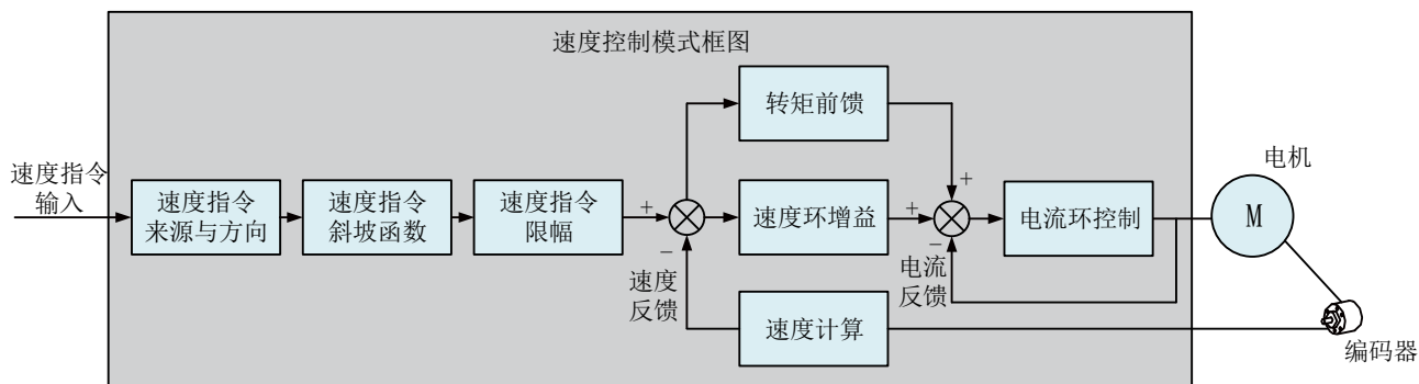
图6-63 速度控制框图
