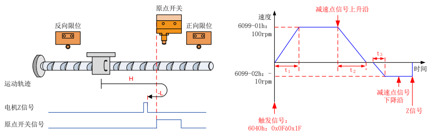
图 4-21 6098h=3 且减速点信号无效模式①
