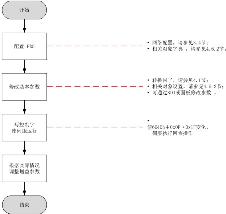
图 4-42 原点回零模式设置流程图举例
