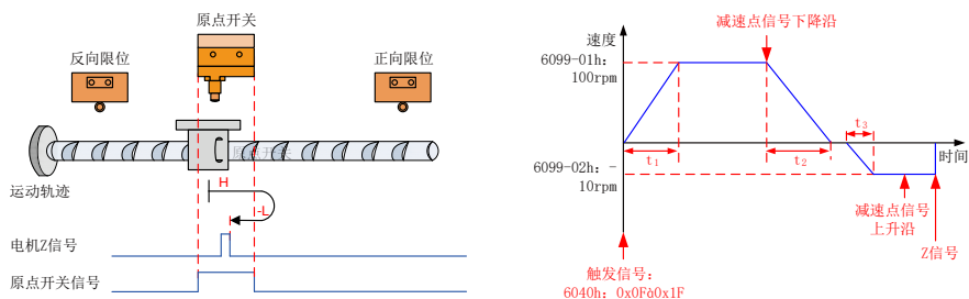
图 4-28 6098h=6 且减速点信号有效模式②
