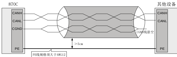
图 2-15 其它设备 CAN 无接地端口
