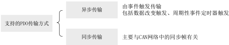
图 3-11 支持的 PDO 传输方式
