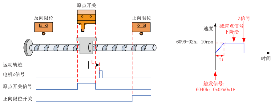
图 4-40 6098h=10 且减速点信号有效模式③
