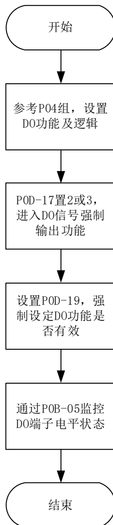
图 5-11 D0 信号强制输出设定步骤示意图
