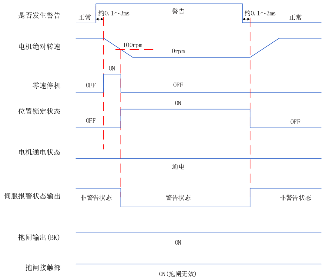
图7-17 需停机类警告时序图
