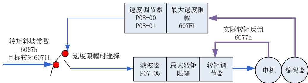
图 7-32 轮廓转矩模式（pt）控制框图
