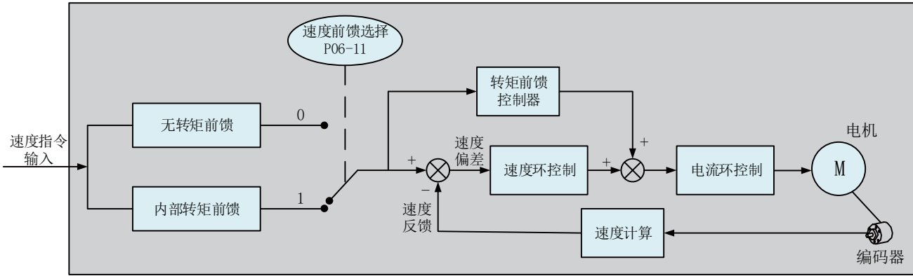
图 9-10 转矩前馈控制操作图
