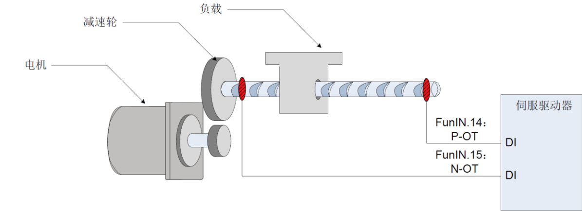
图7-20 限位开关的安装示意图
