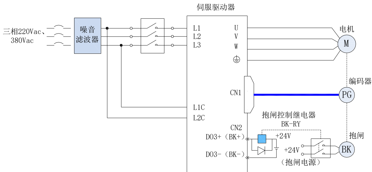
图 7-4 抱闸配线图
