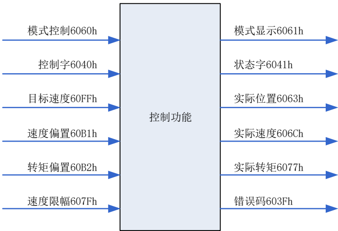
图 7-25 输入输出对象
