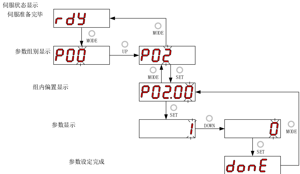
图 5-5 参数设定步骤示意图
