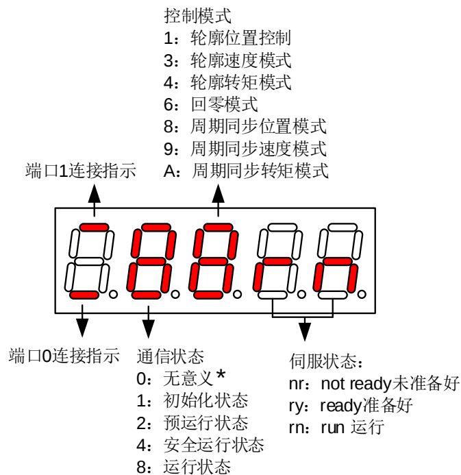
图6-5 状态指示示意图
