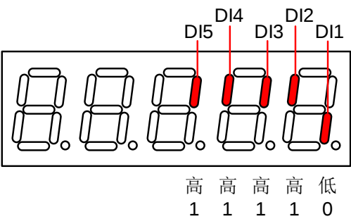
图 5-10 POB-03 对应 DI 电平状态说明
