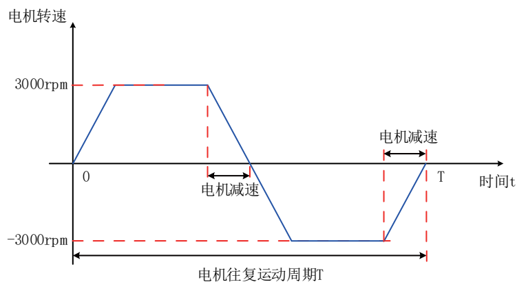
图7-7 外部负载转矩不存在情况下电机速度曲线举例
