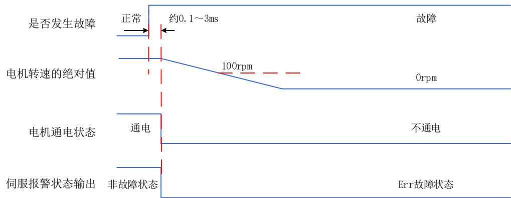
图7-14 故障2时自由停机保持自由运行状态时序图
