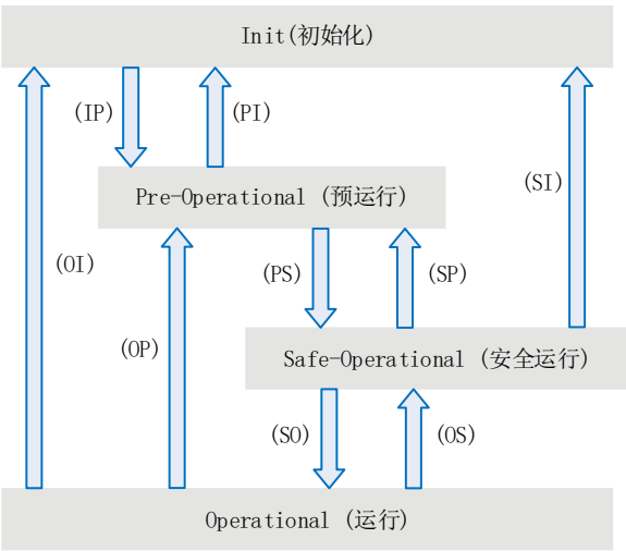
图 6-4 ETherCAT 状态机
