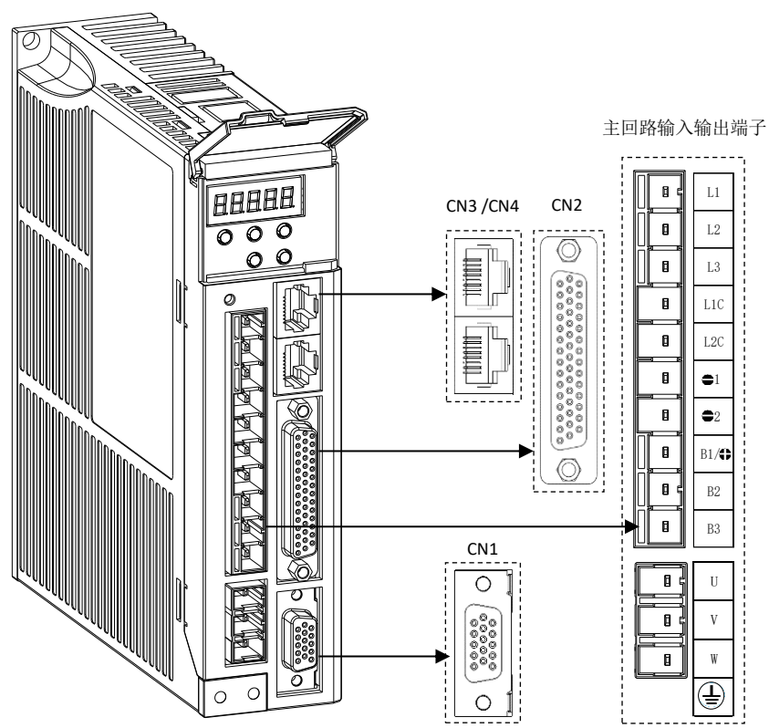
图2-2 伺服驱动器组成
