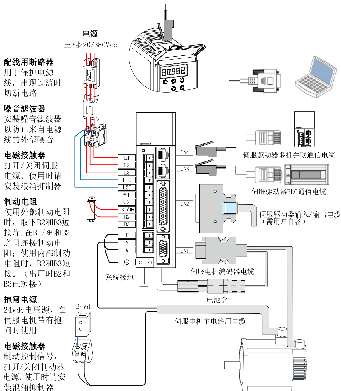
图 2-3 系统配线图举例
