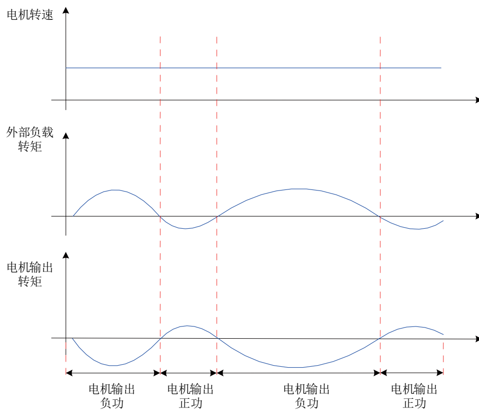
图7-11 外部负载扭矩存在情况下曲线举例
