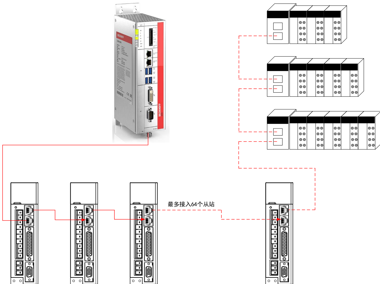
图 6-2 EtherCAT 组网示意图
