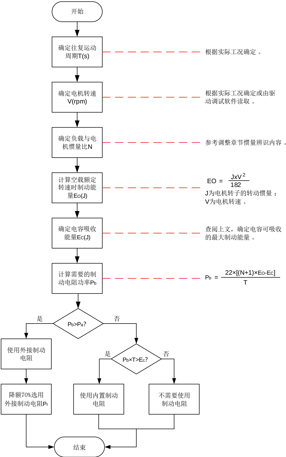
图7-8 制动电阻选型流程图
