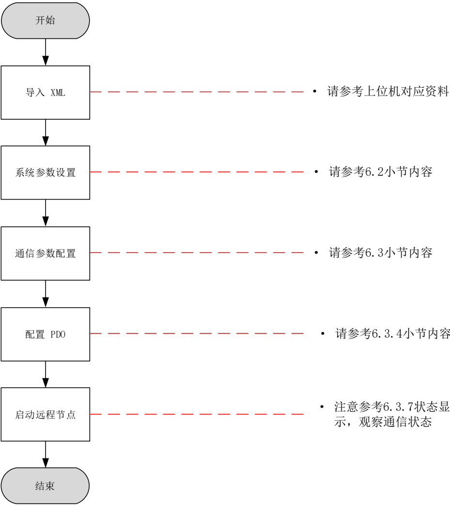
图 6-1 EtherCAT 使用设置流程图
