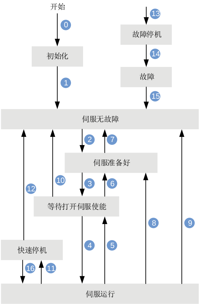
图 7-21 CiA402 状态机切换图
