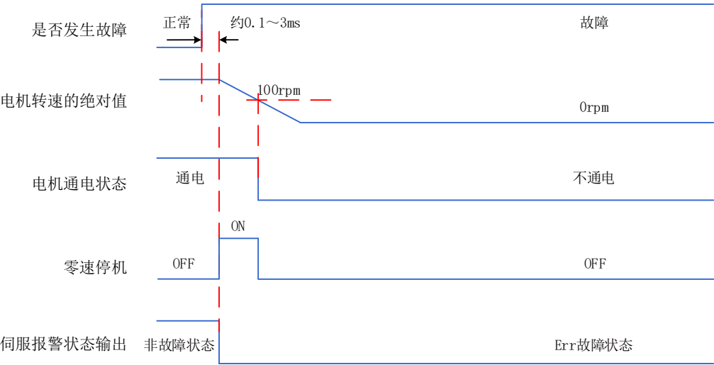
图7-15 故障2（非抱闸）时零速停机保持自由运行状态时序图
