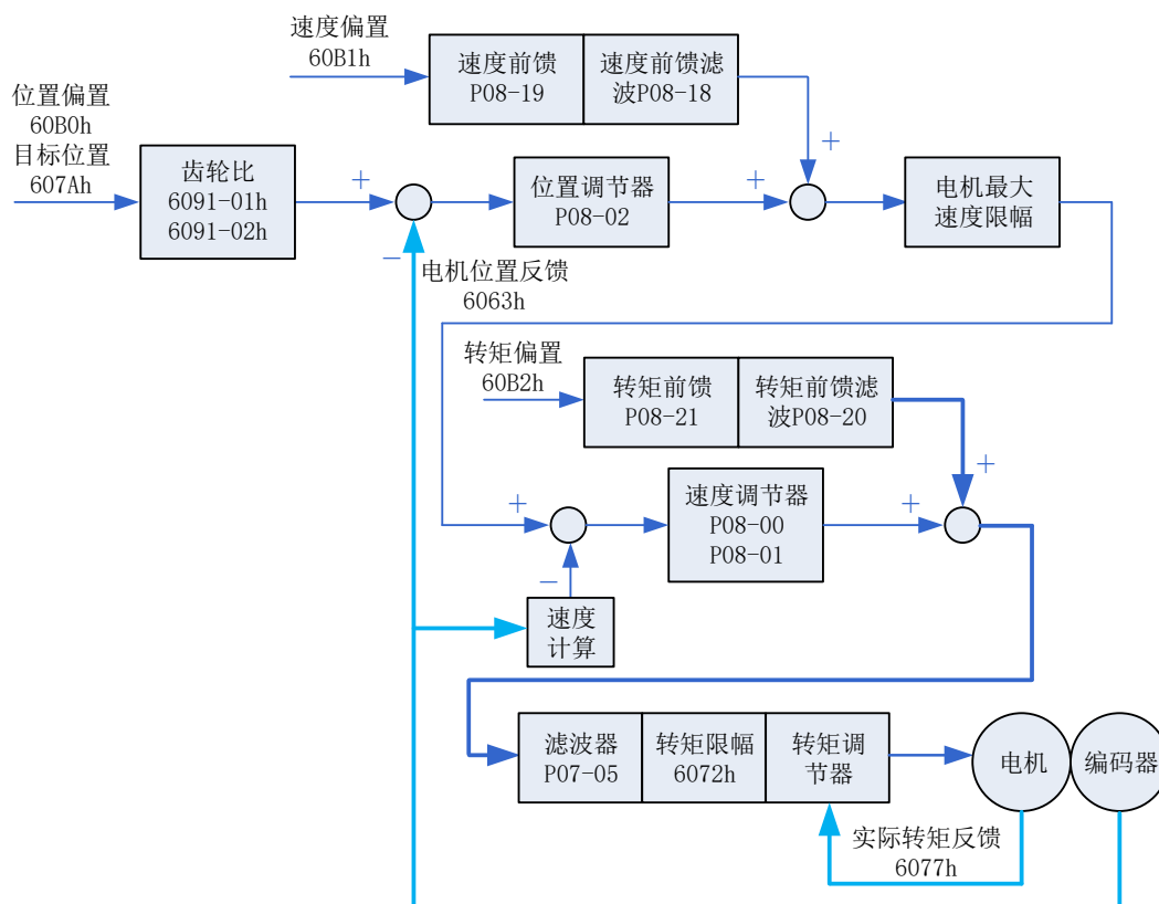
图 7-22 同步周期位置配置框图
