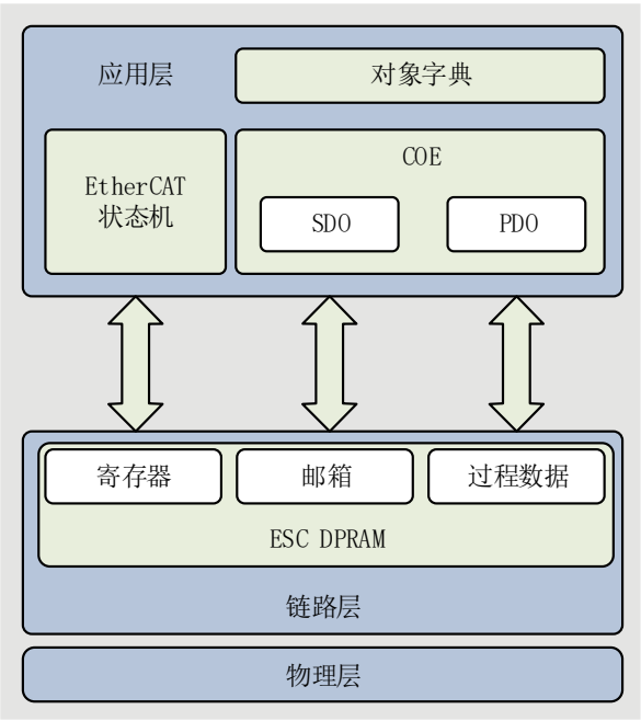
图 6-3 基于 CANOpen 应用层的 EtherCAT 通信结构
