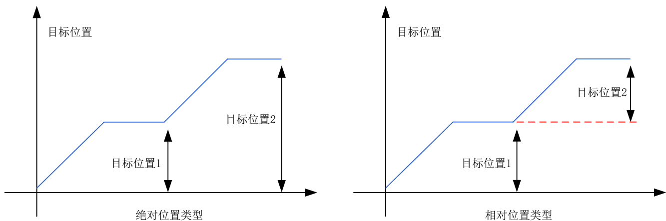
图 7-30 绝对位置指令与相对位置指令的区别
