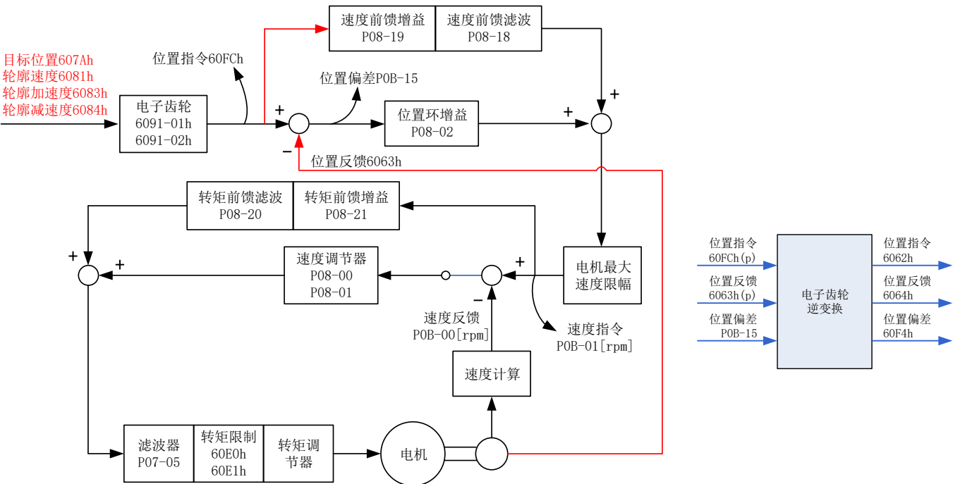
图 7-26 轮廓位置模式 (pp) 控制框图
