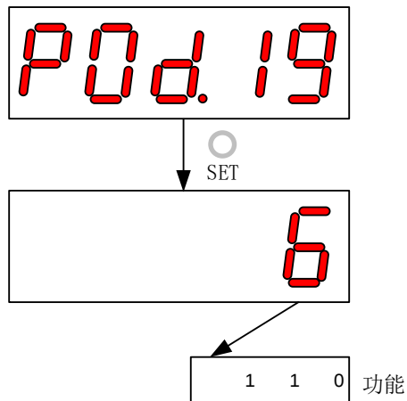
图 5-12 P0D-19 设定含义说明
