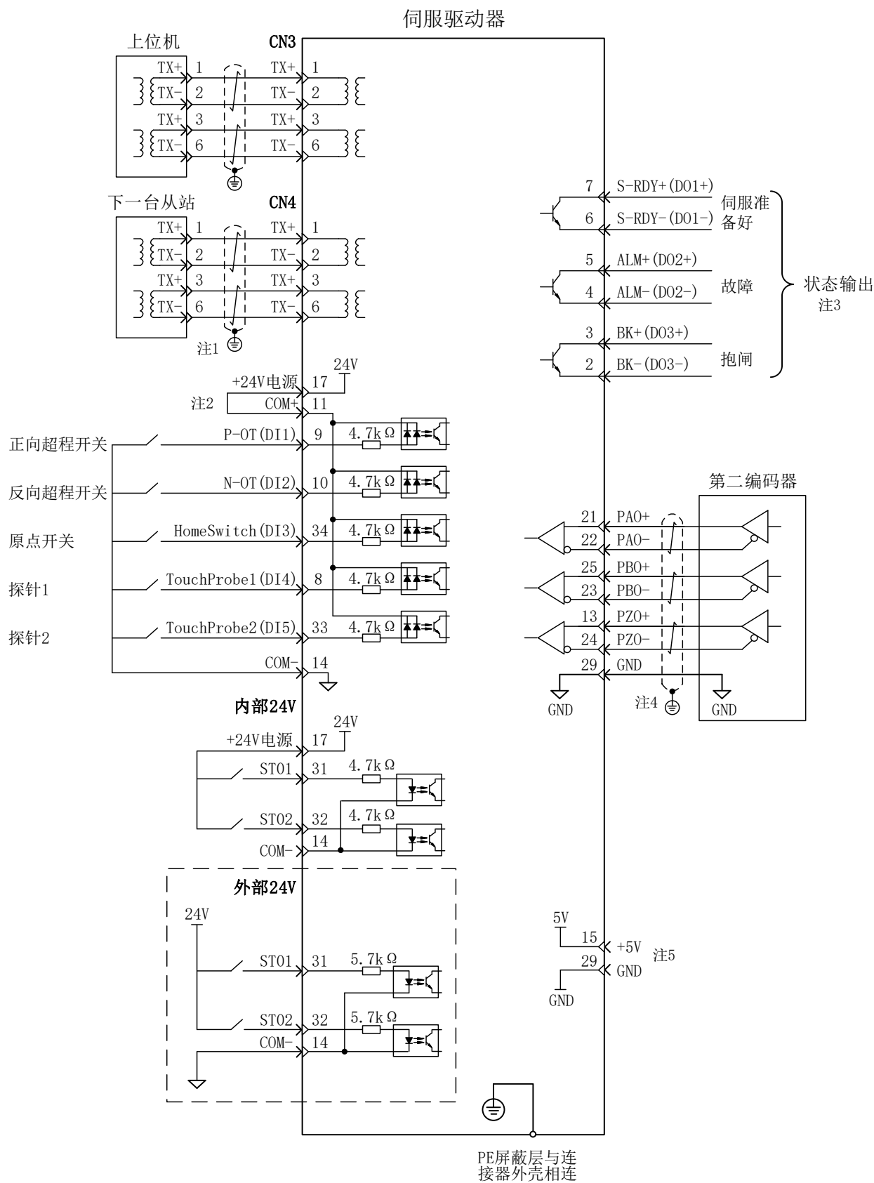
图 4-20 总线配线示意图
