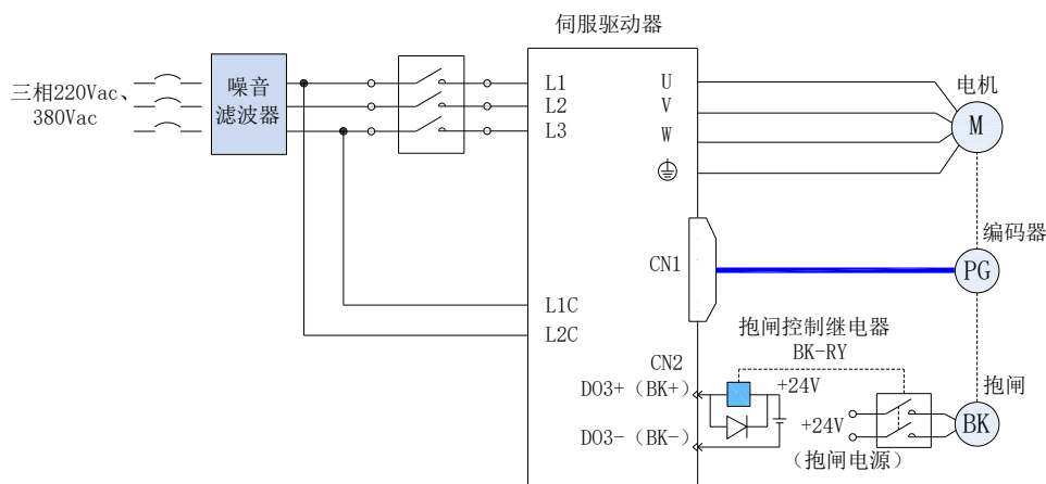
图4-10 抱闸配线图
