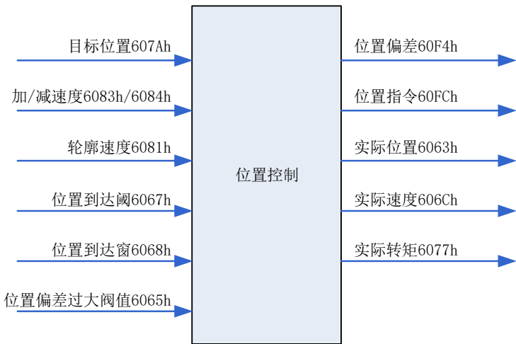
图 7-27 轮廓位置模式 (pp) 输入输出框图
