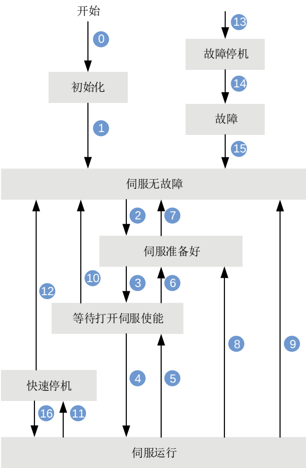
图6-6 CiA402状态机切换图
