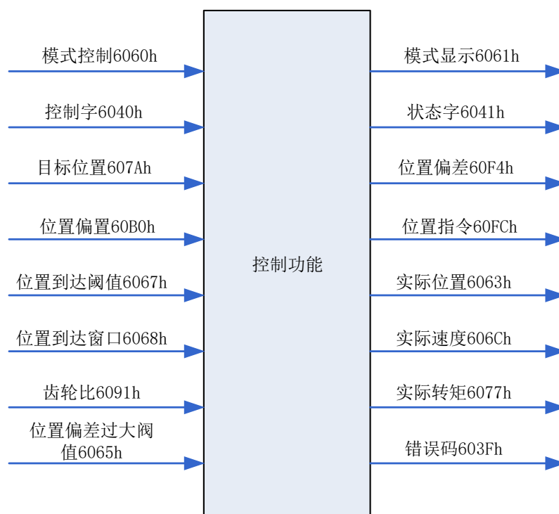
图 7-23 输入输出对象
