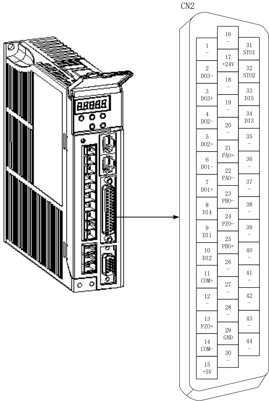
图4-8 驱动器控制回路端子连接器引脚分布图
