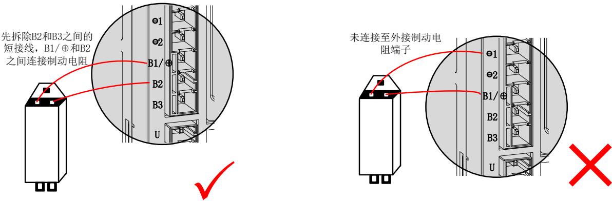
图7-9 外接制动电阻连接示意图
