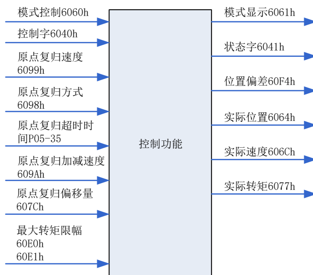
图 7-34 输入输出对象
