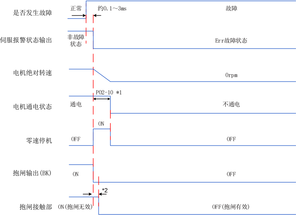
图7-16 故障2（带抱闸）时零速停机方式自由停机状态时序图
