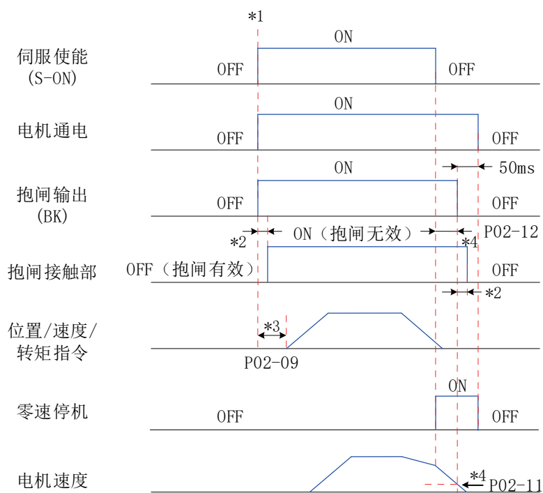
图 7-6 电机旋转时抱闸时序图
