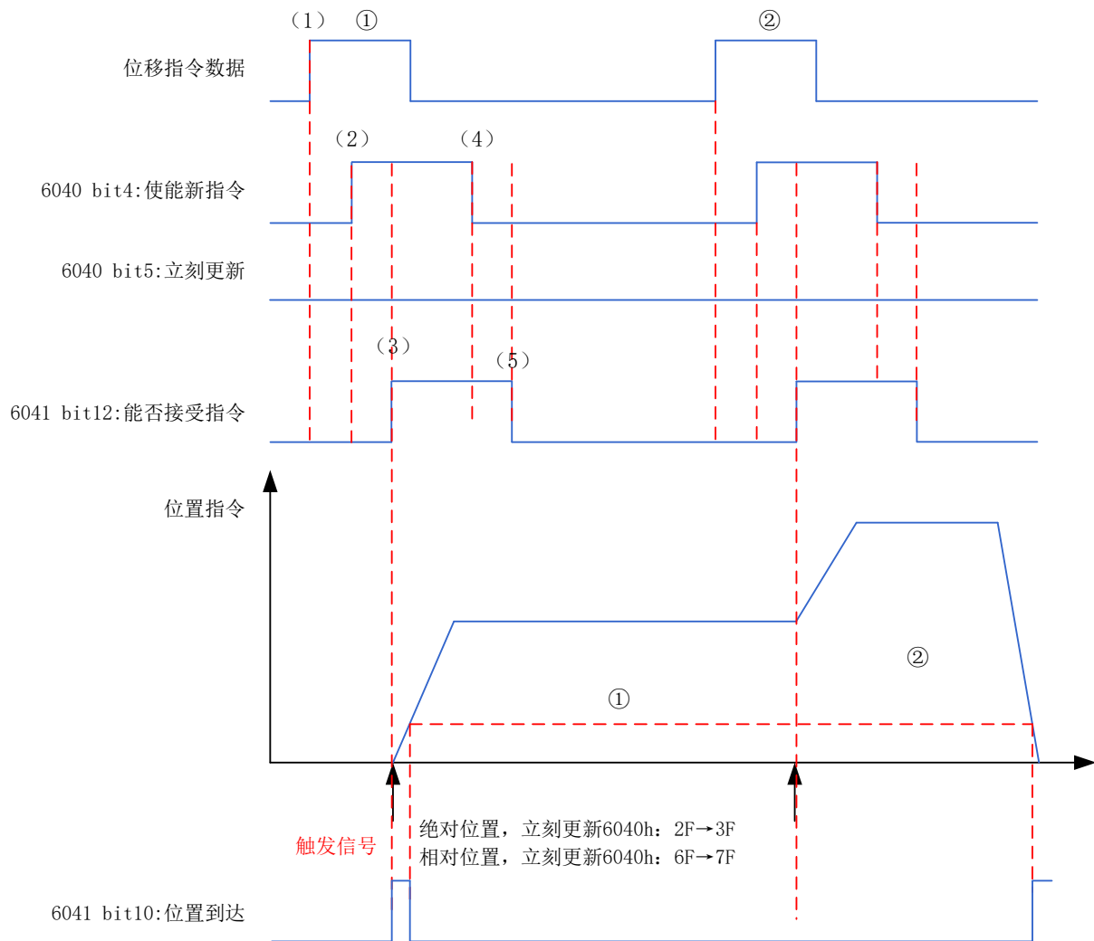
图 7-28 立刻更新型时序图与电机运行曲线
