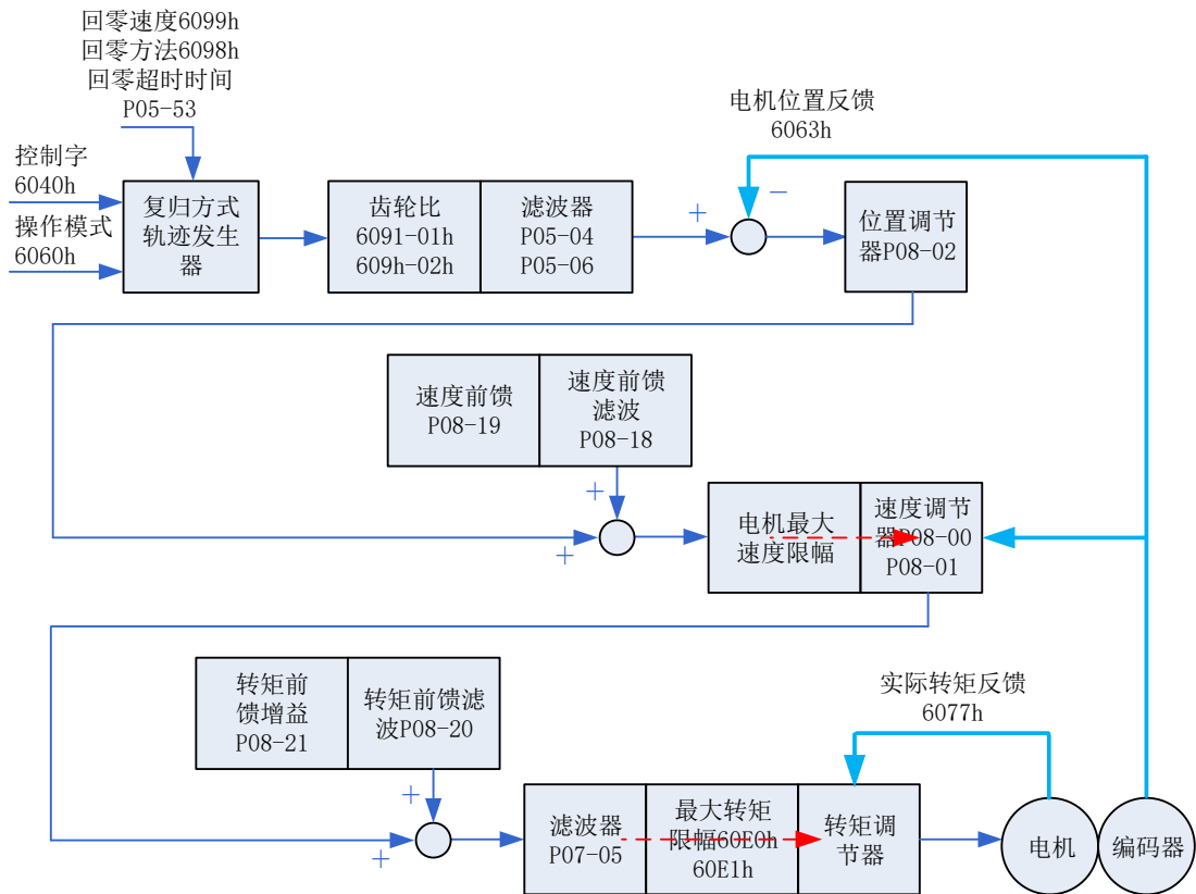
图 7-33 原点回归模式控制框图
