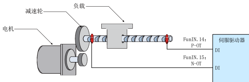
图 7-43 限位开关的安装示意图
