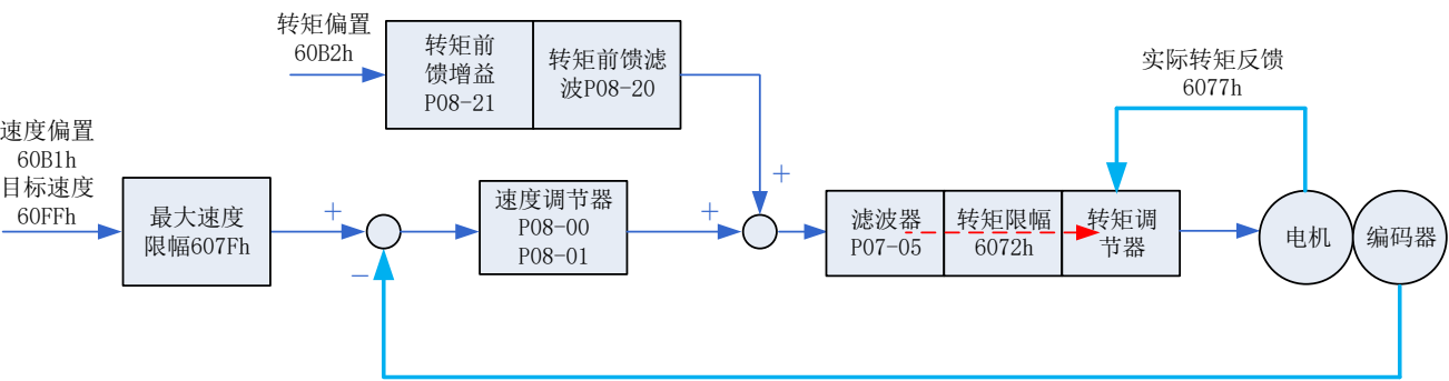
图 7-24 同步周期速度模式（csv）配置框图
