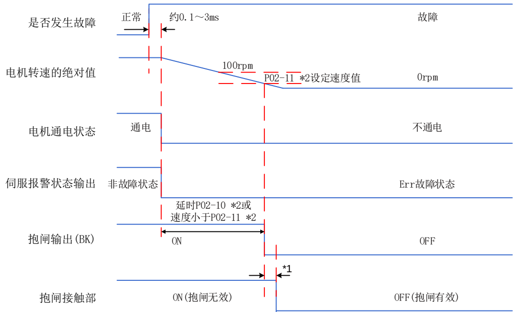
图7-13 故障1时自由停机保持自由运行状态时序图
