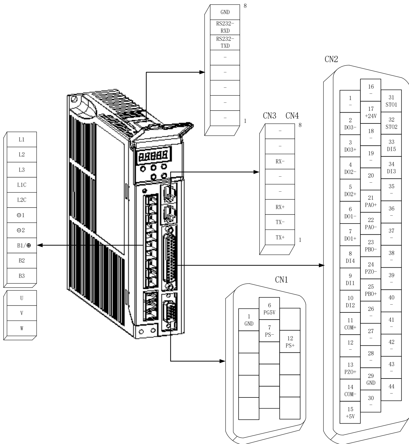
图4-1 伺服驱动器端子引脚分布图
