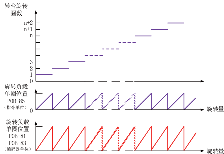
图 7-41 旋转负载单圈位置与转台位置对应关系示意图
