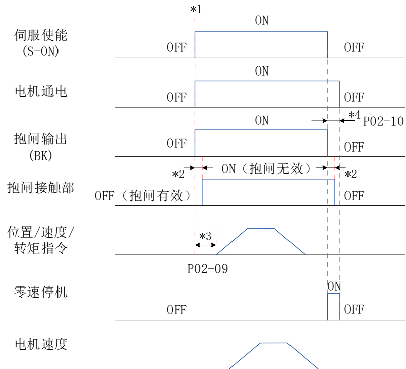
图 7-5 电机静止时抱闸时序图
