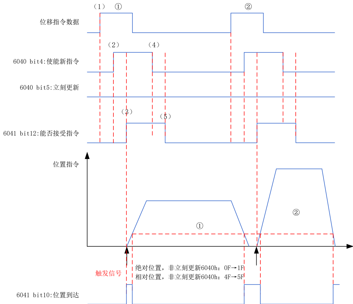
图 7-29 非立刻更新型时序图与电机运行曲线
