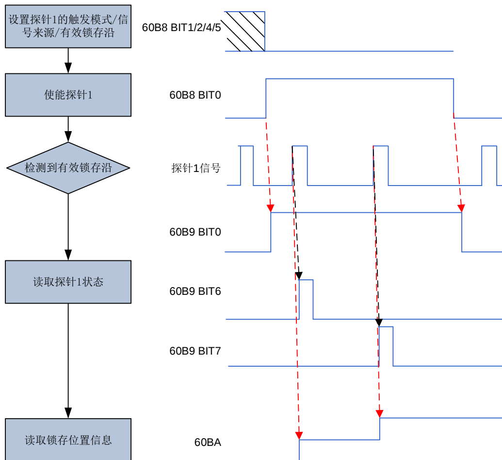
图 7-35 探针使用步骤图示
