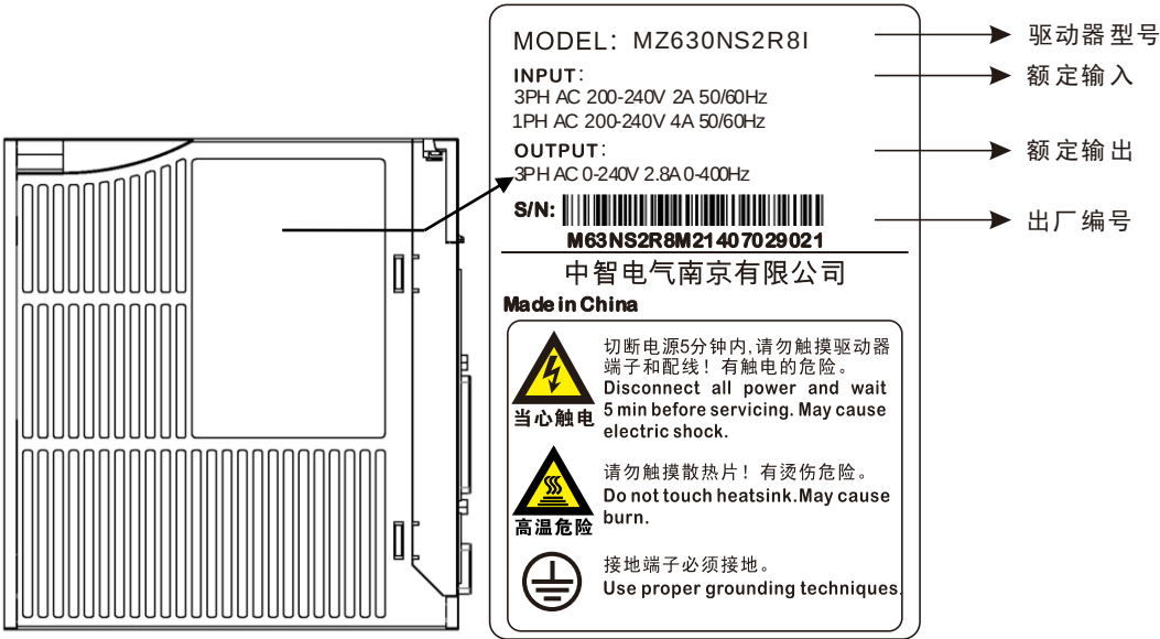
图2-1 驱动器命名与规则
