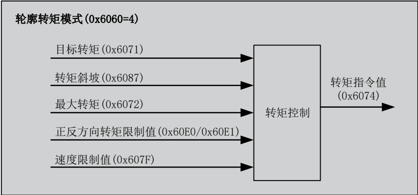
图 7-32 轮廓转矩模式（pt）控制框图
