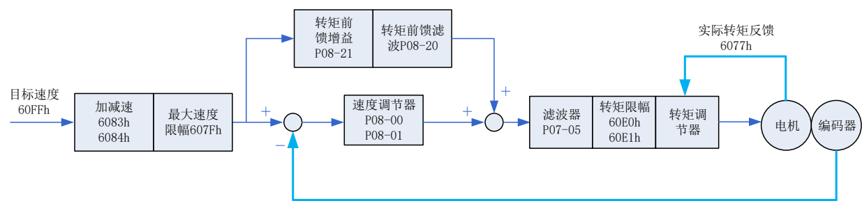
图 7-31 轮廓速度模式（pv）控制框图
