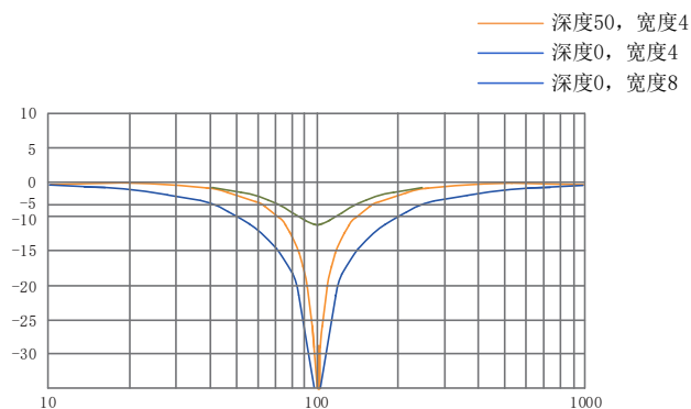
图 9-15 陷波器频率特性
