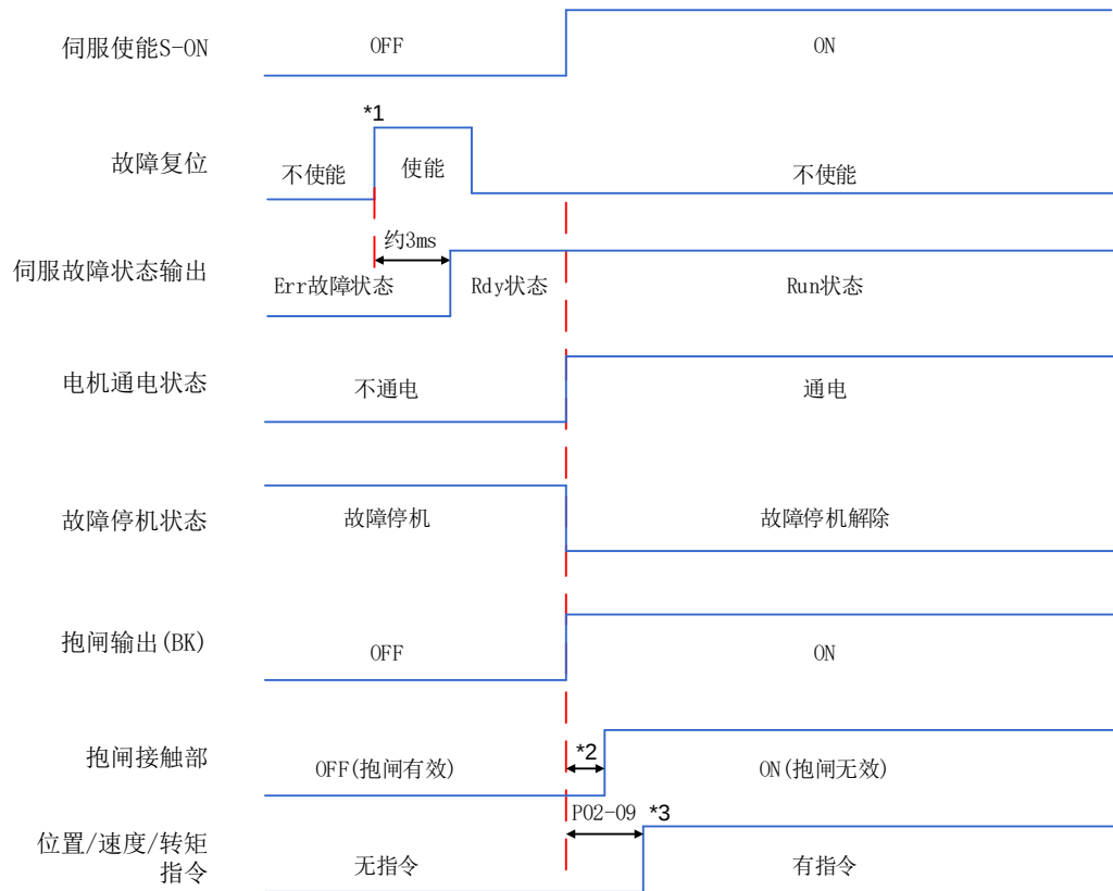
图7-19 故障复位时序图
