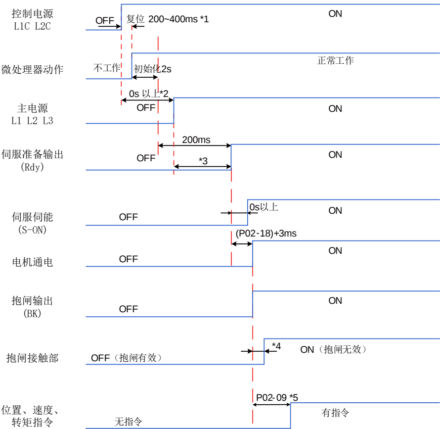
图7-12 电源接通时序图
