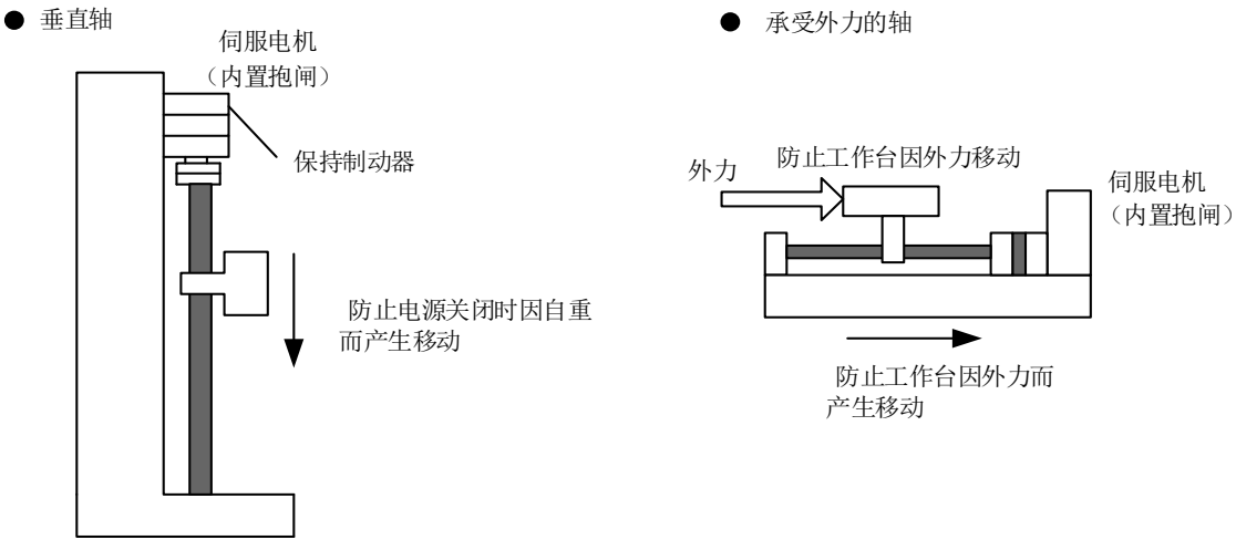
图 7-3 抱闸应用示意图
