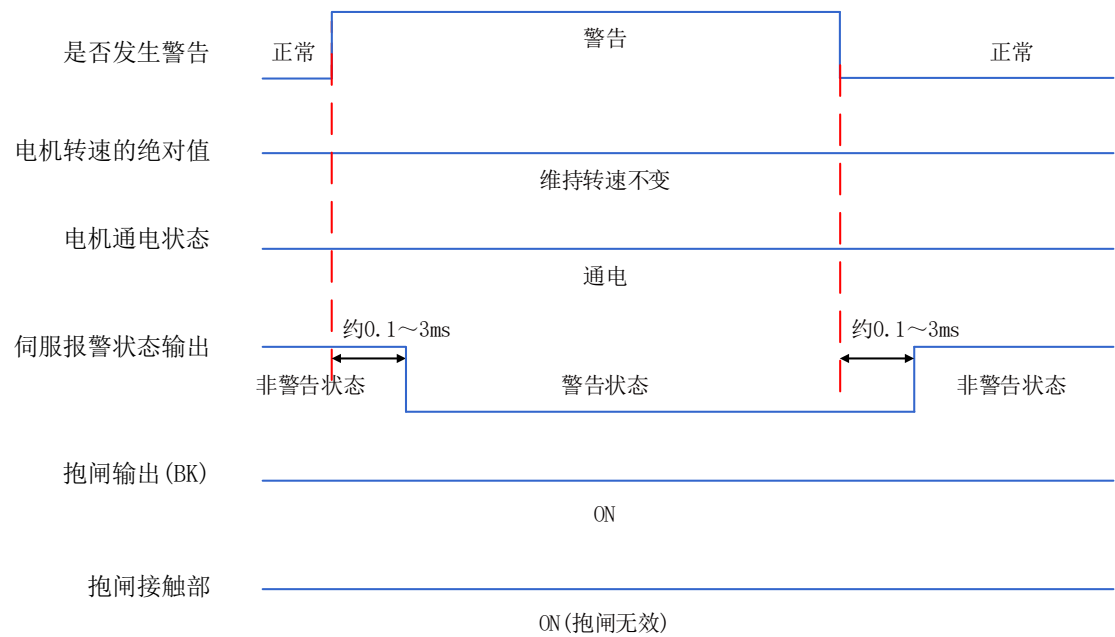
图7-18 非停机警告时序图
